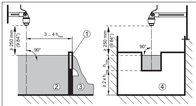
Fig. 13: Flowmeting met rechthoekig overstortschot: h_{max} = max. vulling van het rechthoekig overstortschot
