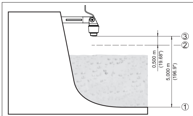
Fig. 20: Parametrevoorbeeld min.-/max.-inregeling
