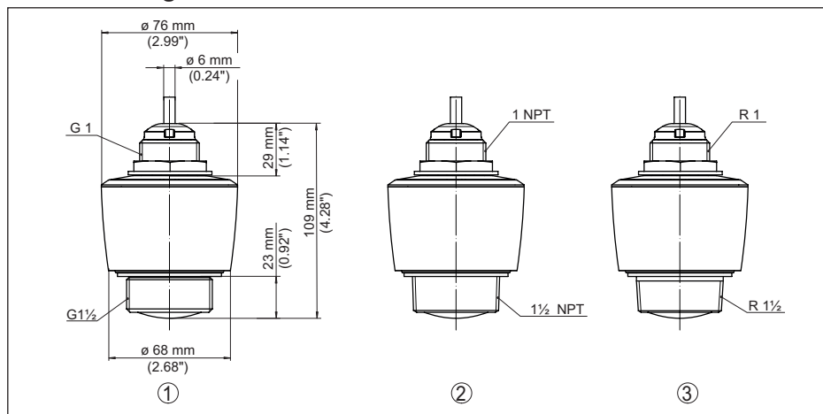
Fig. 29: Afmetingen VEGAPULS C 21
