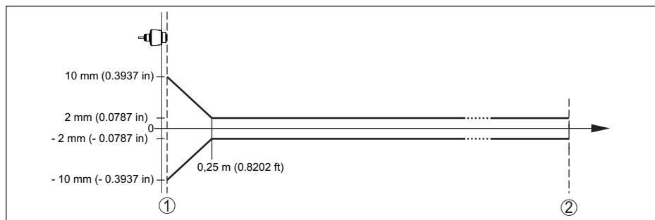
Fig. 27: Meetnauwkeurigheid onder referentiecondities 10)
