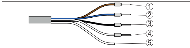
Fig. 18: Aderbezetting vast aangesloten aansluitkabel
