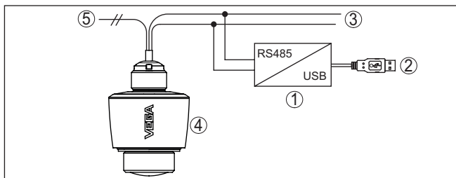
Fig. 4: Aansluiting van de PC op de signaalkabel
