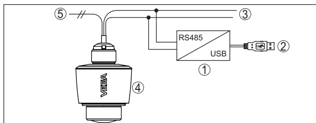
Fig. 23: Aansluiting van de PC op de signaalkabel
