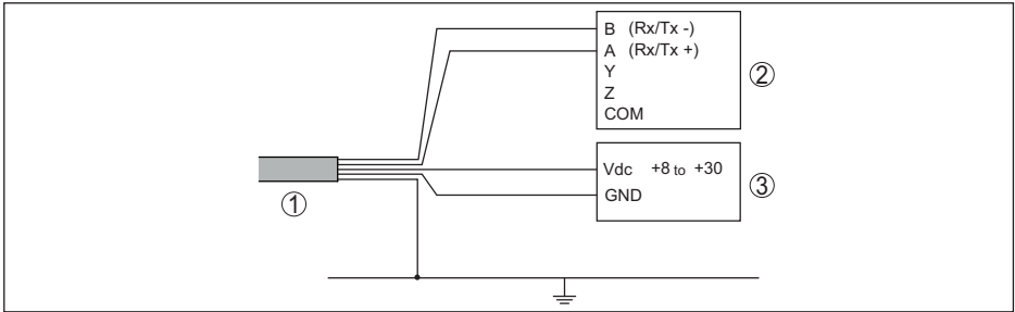
Fig. 28: Aansluiting van de VEGAPULS C 21 op RTU Fisher ROC 809
