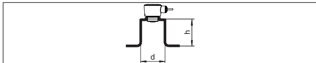
Fig. 13: Montage de la rehausse en cas de dimensions de rehausse différente
