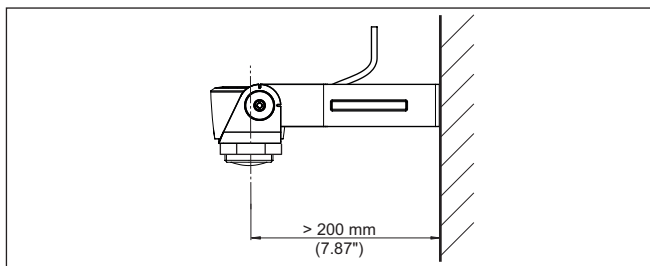
Fig. 6: Montage par une équerre de montage
