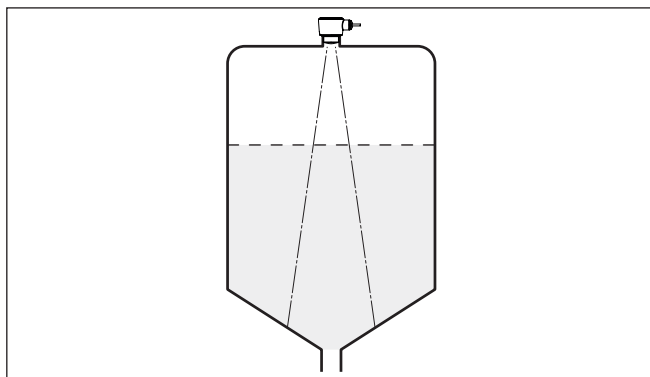
Fig. 9: Montage du capteur radar dans des cuves à fond conique
