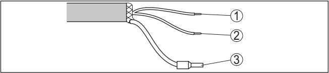
Fig. 19: Affectation des conducteurs du câble de raccordement raccordé de façon fixe
