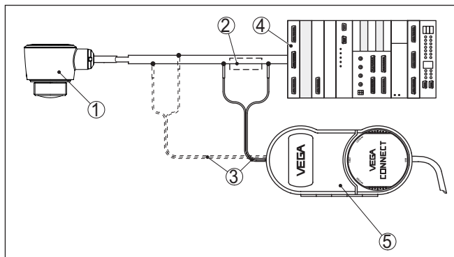
Fig. 24: Raccordement du PC à la ligne signal
