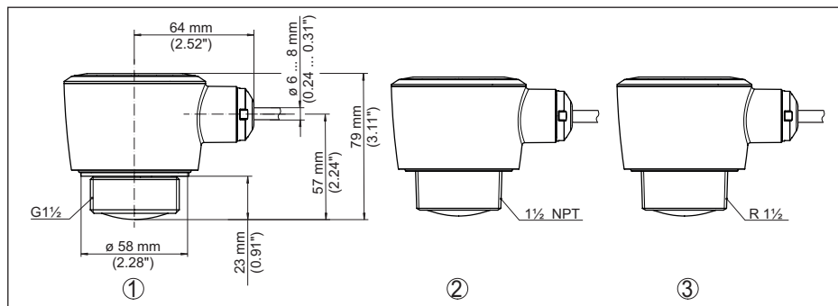
Fig. 31: Encombrement VEGAPULS C 22
