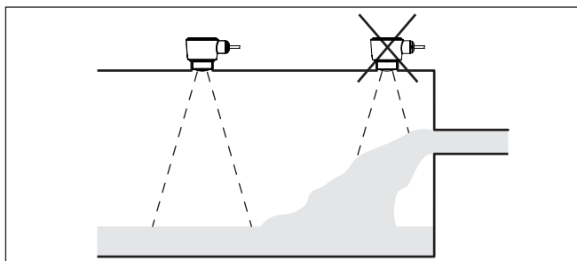
Fig. 11: Montage du capteur radar en présence d'un flux de produit
