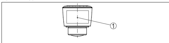
Fig. 7: Sens de la polarisation
