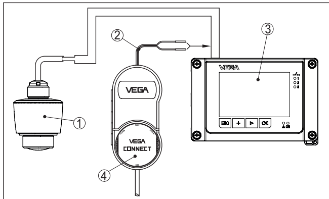
Fig. 25: Raccordement du PC à l'unité de commande VEGAMET
