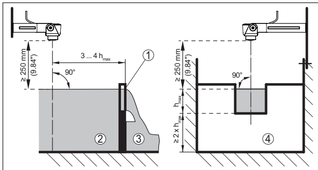
Fig. 18: Mesure du débit avec déversoir rectangulaire: h_{max} = remplissage max. du déversoir rectangulaire
