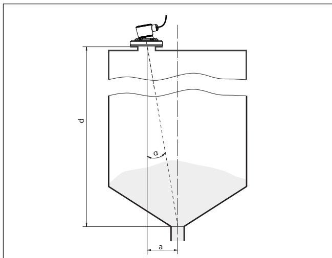
Fig. 16: Proposition pour un montage après orientation VEGAPULS C 22
