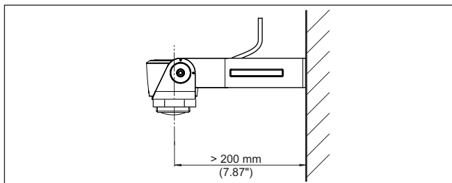
Fig. 5: Montage par une équerre de montage
