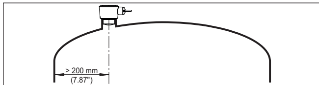
Fig. 7: Montage du capteur radar dans une cuve à toit bombé
