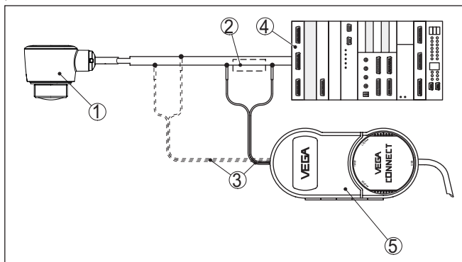
Fig. 3: Raccordement du PC à la ligne signal
