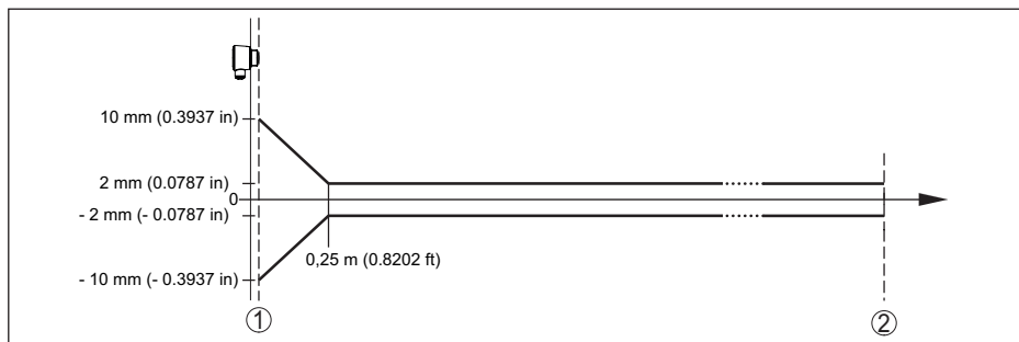
Fig. 31: Écart de mesure sous conditions de référence 10)
