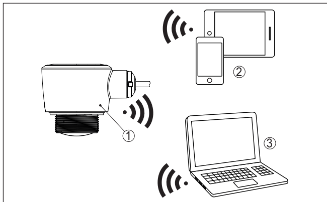
Fig. 2: Connexion sans fil aux unités de réglage standard avec Bluetooth intégré LE
