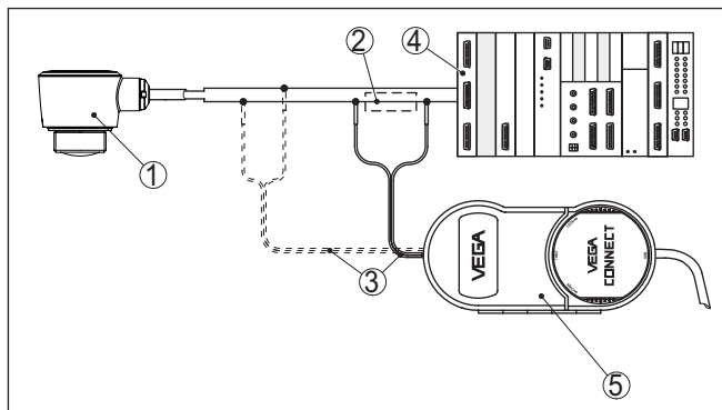
Fig. 25: Raccordement du PC à la ligne signal
