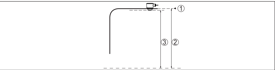
Fig. 29: Données relatives à la grandeur d'entrée
