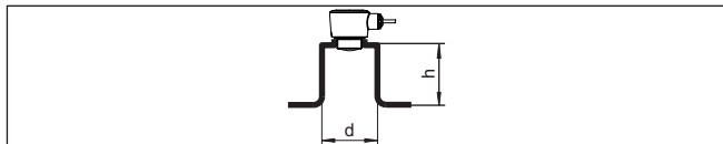
Fig. 12: Montage de la rehausse en cas de dimensions de rehausse différente
