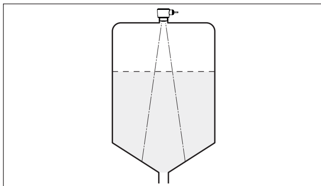
Fig. 8: Montage du capteur radar dans des cuves à fond conique
