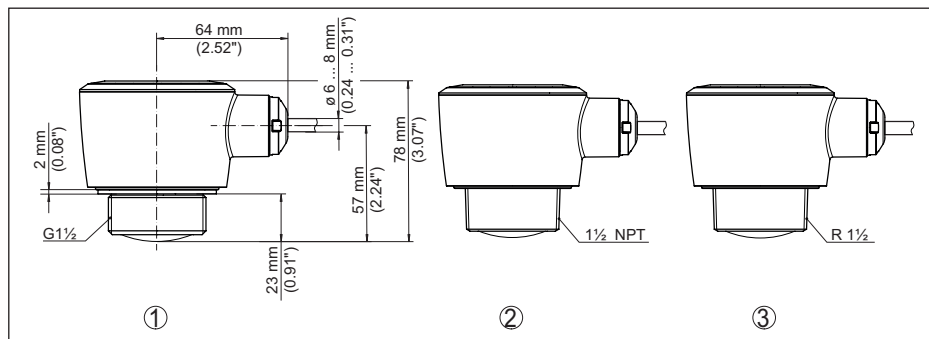
Fig. 32: Encombrement VEGAPULS C 22
