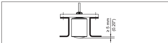
Fig. 10: Montage sur rehausse du VEGAPULS C 23 recommandé
