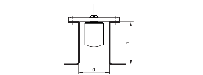
Fig. 11: Montage de la rehausse en cas de dimensions de rehausse différente
