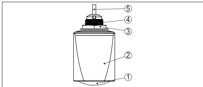
Fig. 1: Composants du VEGAPULS C 23
