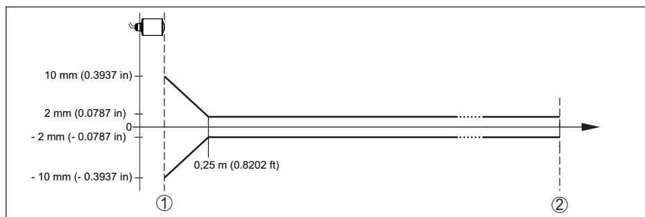
Fig. 30: Écart de mesure sous conditions de référence 8)
