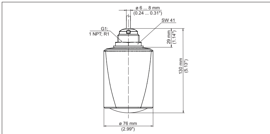
Fig. 31: Encombrement VEGAPULS C 23
