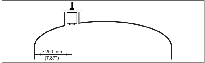
Fig. 6: Montaje del sensor en tapas de depósitos redondas
