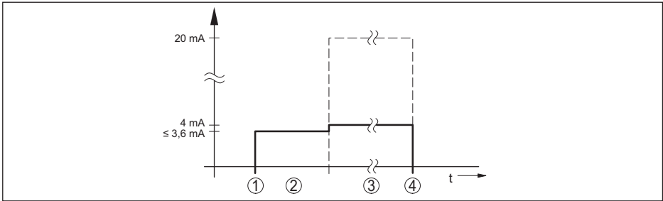
Fig. 28: Tiempo de aceleración y salida del valor de medición
