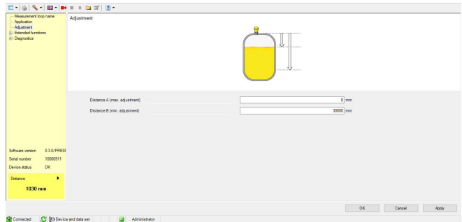
Fig. 26: Ejemplo de una vista DTM
