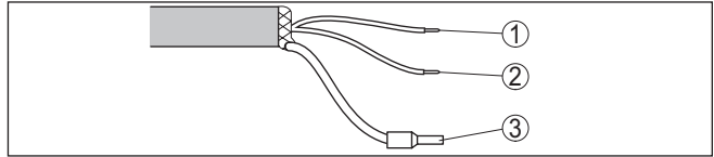
Fig. 19: Dotación de conductores, cable de conexión de conexión fija
