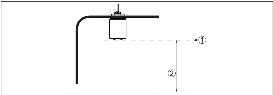
Fig. 29: Datos para la magnitud de entrada
