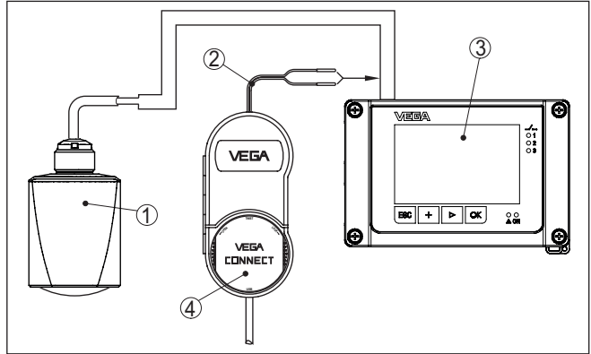
Fig. 25: Conexión del PC al controlador VEGAMET
