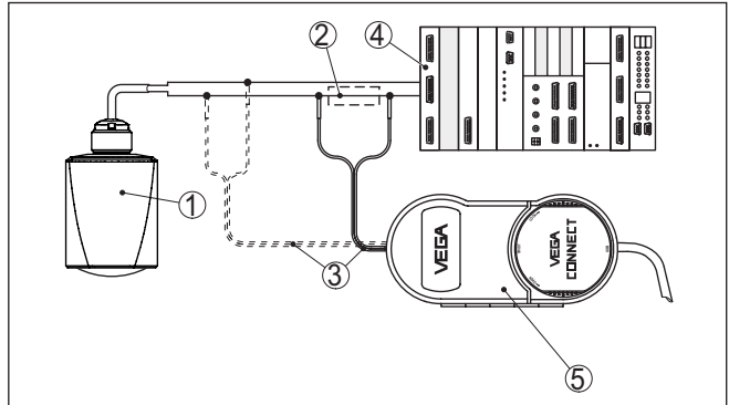
Fig. 3: Conexión del PC a la línea de señal
