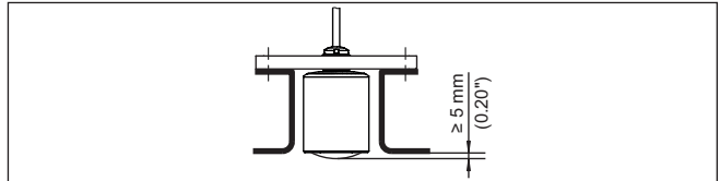
Fig. 10: Montaje recomendado en tubuladura del VEGAPULS C 23
