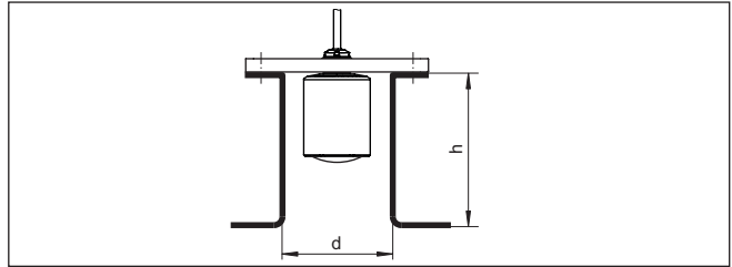
Fig. 11: Montaje de tubuladuras con medidas divergentes
