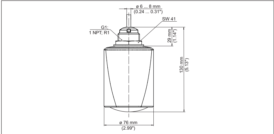
Fig. 31: Medidas VEGAPULS C 23
