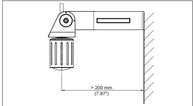
Fig. 4: Montaje a través de un brazo de soporte
