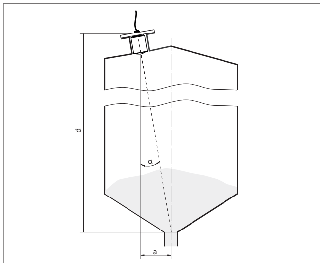
Fig. 15: Propuesta de montaje después de la orientación VEGAPULS C 23
