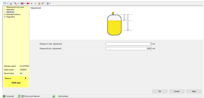
Fig. 23: Ejemplo de una vista de DTM - Configuración ajuste del sensor
