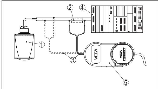
Fig. 24: Conexión del PC a la línea de señal
