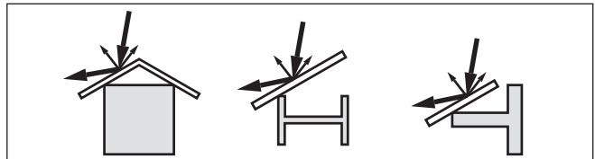
Fig. 12: Tapar los perfiles lisos con pantallas dispersoras
