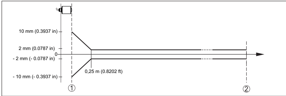
Fig. 30: Error de medición bajo condiciones de referencia 8)
