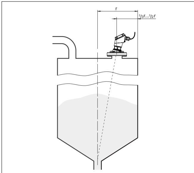
Abb. 13: Montageposition und Ausrichtung
