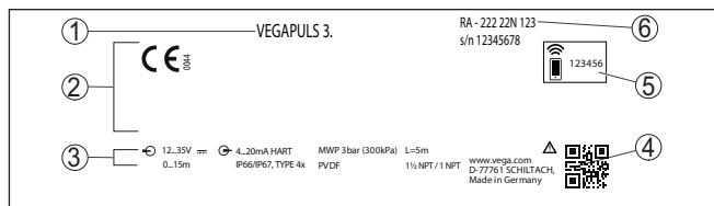
Abb. 2: Aufbau des Typschildes (Beispiel)
