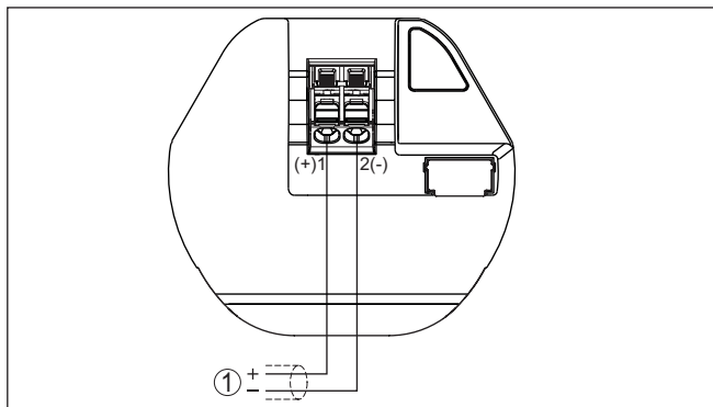
Abb. 19: Anschlussraum VEGAPULS 11
