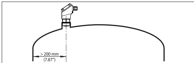
Abb. 5: Montage des Radarsensors an runden Behälterdecken
