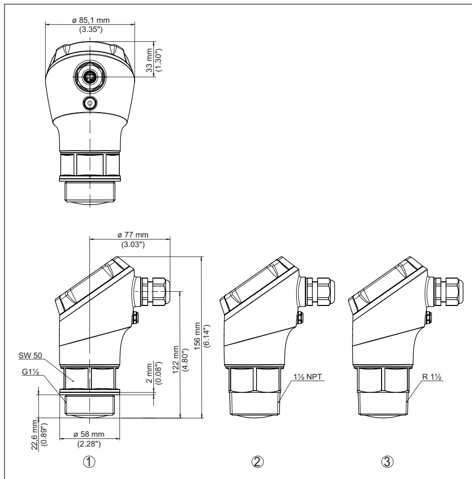
Abb. 28: Maße VEGAPULS 11
