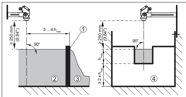
插图. 14: 用矩形槽测量流量： h_{max} = 矩形槽的最大注水高度
