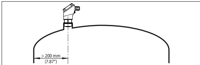
插图. 5: 将雷达传感器安装在圆形容器盖面上
