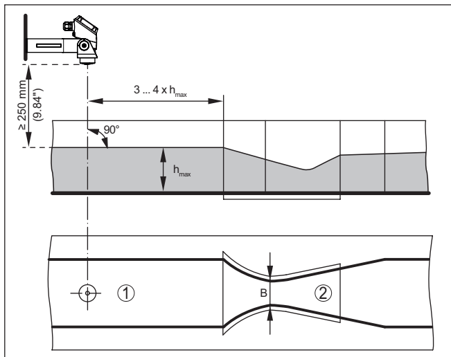
插图. 15: 用卡发基-文丘里槽来测量流量： h_{max} = 水槽的最大灌装量；B = 水槽的最大收缩率
