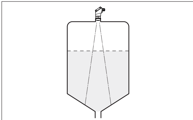
插图. 6: 将雷达传感器安装到带有锥形底部的容器上
