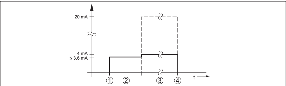
插图. 24: 启动时间和测量值的输出
