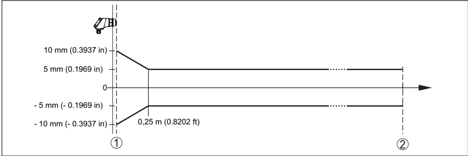
插图. 25: 在基准条件下的测量偏差 9)
