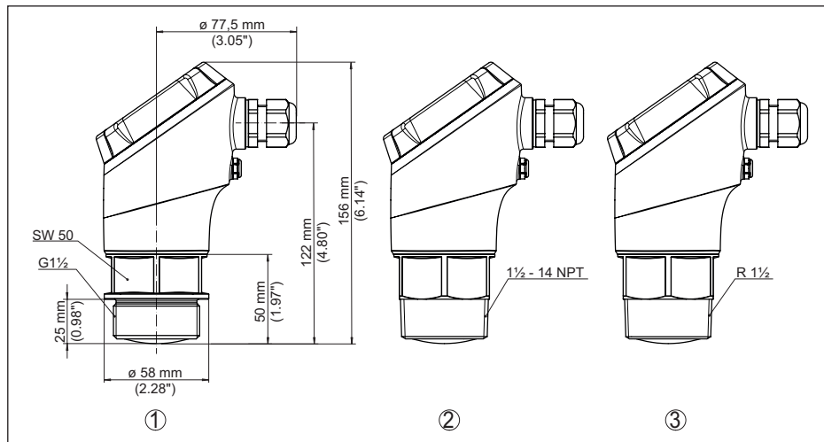
插图. 26: VEGAPULS 11 的尺寸
