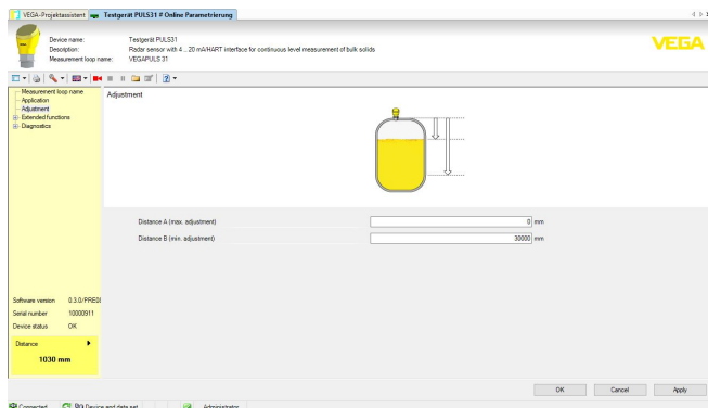
插图. 21: DTM 视图举例 - 调试 传感器调整
