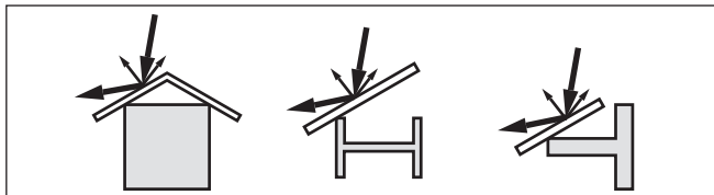
插图. 11: 用散射挡板来覆盖光滑的型材
