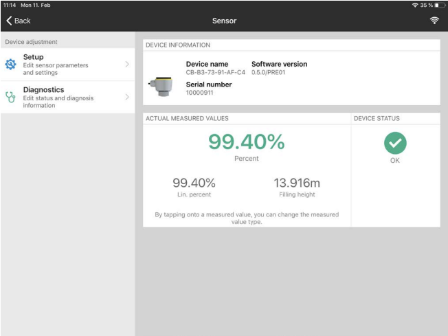
插图. 19: App 应用程序视图举例 - 调试 调整
