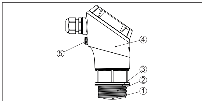
插图. 1: VEGAPULS 11的部件
