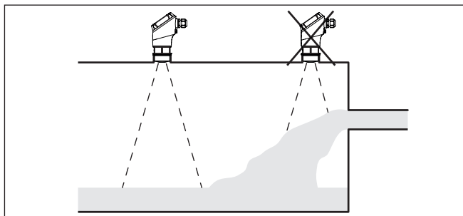
Fig. 9: Montage du capteur radar en présence d'un flux de produit
