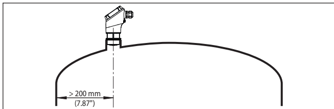
Fig. 6: Montage du capteur radar dans une cuve à toit bombé
