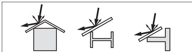
Fig. 11: Recouvrir les obstacles lisses par des déflecteurs
