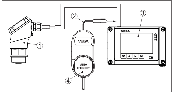
Fig. 26: Raccordement du PC à l'unité de commande VEGAMET
