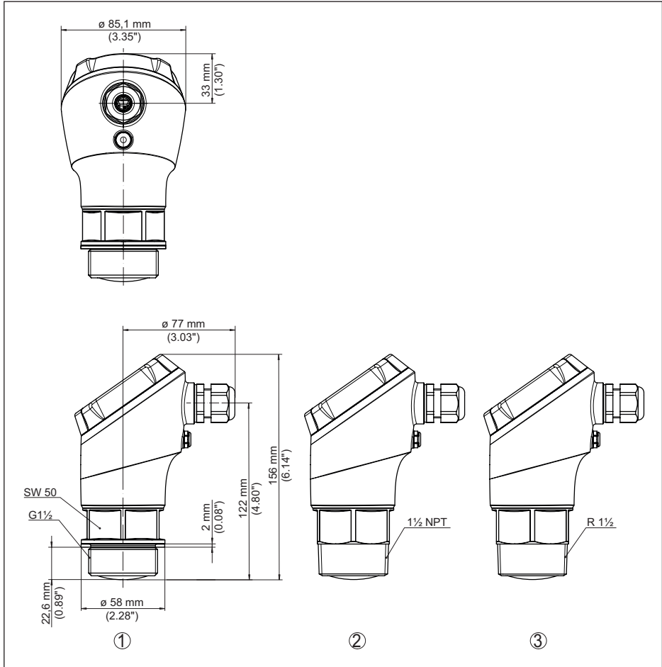
Fig. 32: Encombrement VEGAPULS 21
