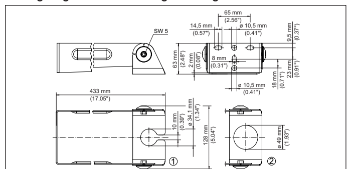
Abb. 26: Montagebügel zur Wandmontage - Ausleger 200 mm
