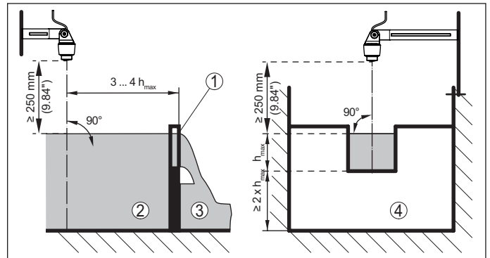
Abb. 10: Durchflussmessung mit Rechtecküberfall: h_{max} = \text{max. Befüllung des Rechtecküberfalls}
