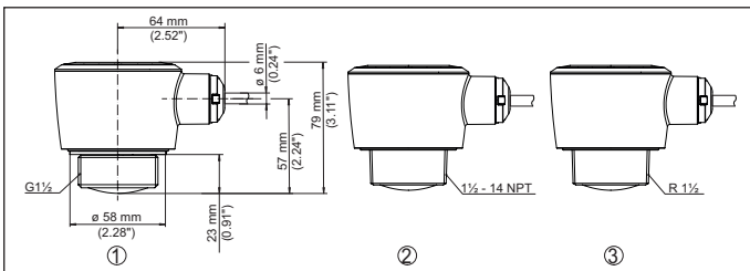
Abb. 22: Maße VEGAPULS C 22
