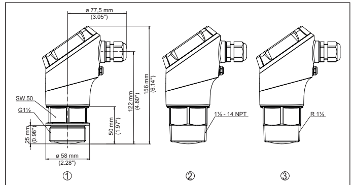
Abb. 24: Maße VEGAPULS 11, 21, 31
