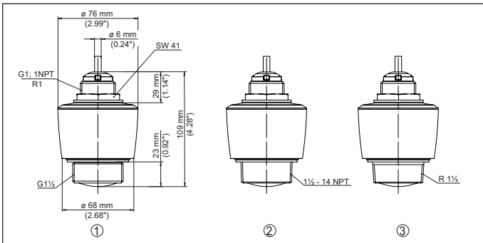
Abb. 21: Maße VEGAPULS C 11, C 21
