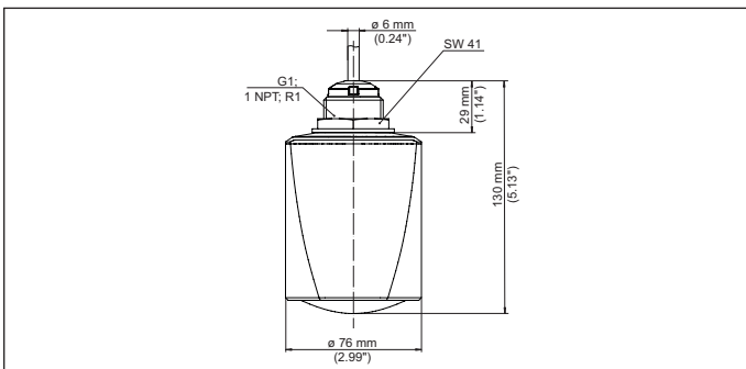
Abb. 23: Maße VEGAPULS C 23
