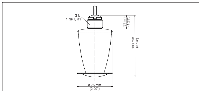
Abb. 23: Maße VEGAPULS C 23
