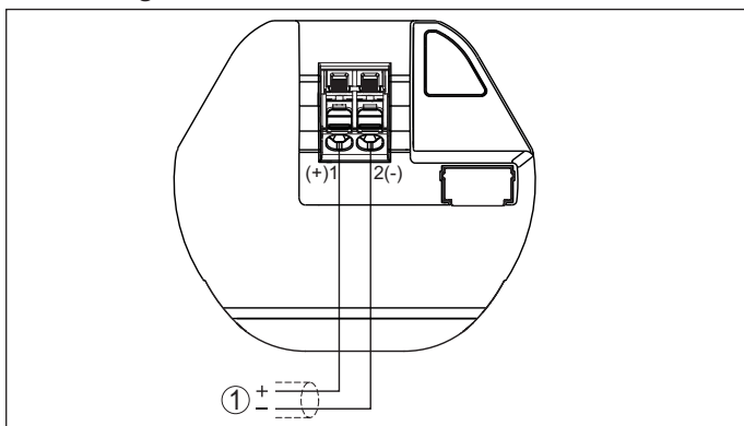
Abb. 13: Anschlussraum VEGAPULS
