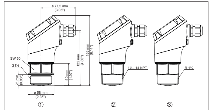
Abb. 24: Maße VEGAPULS 11, 21, 31
