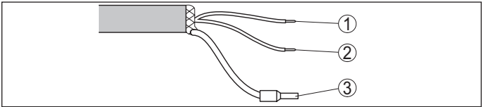
Abb. 14: Aderbelegung fest angeschlossenenes Anschlusskabel
