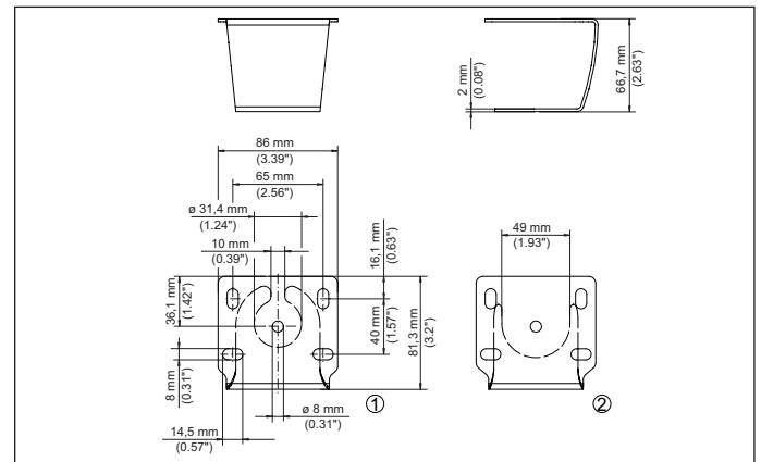
Abb. 25: Montagebügel zur Deckenmontage
