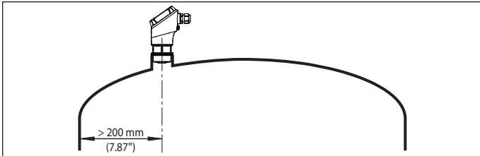
Abb. 6: Montage des Radarsensors an runden Behälterdecken
