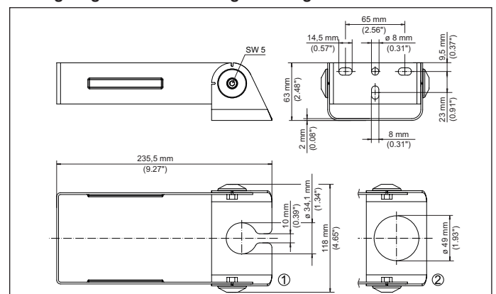
Abb. 26: Montagebügel zur Wandmontage - Ausleger 200 mm
