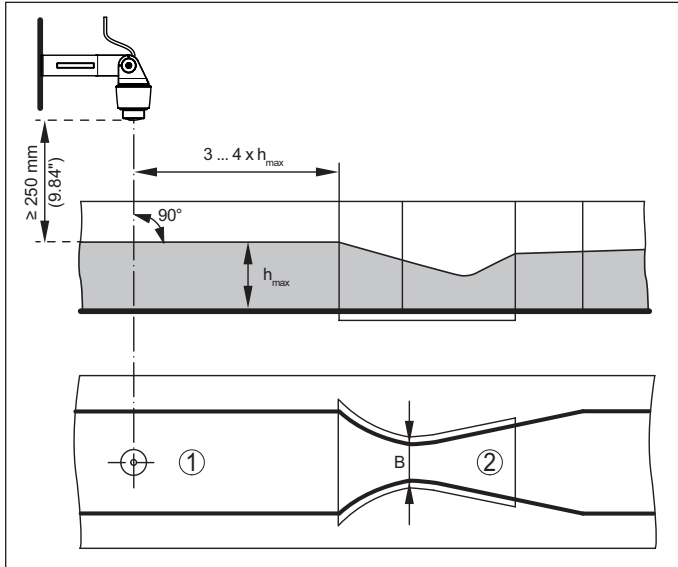
Abb. 11: Durchflussmessung mit Khafagi-Venturirinne: h_{max} = max. Befüllung der Rinne; B = größte Einschnürung der Rinne
