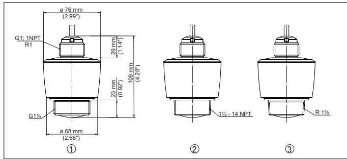
Abb. 21: Maße VEGAPULS C 11, C 21
