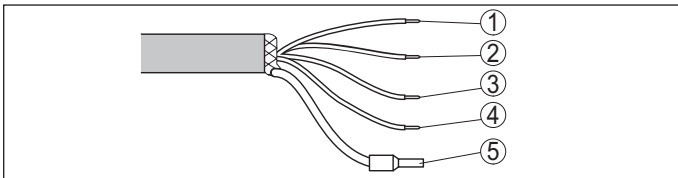
Abb. 17: Aderbelegung fest angeschlossenes Anschlusskabel
