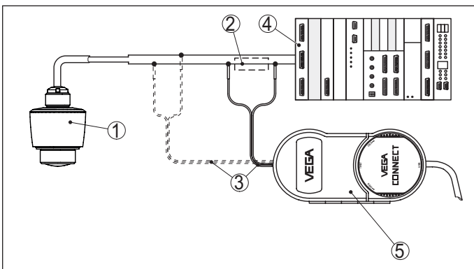
Abb. 19: Anschluss des PCs an die Signalleitung
