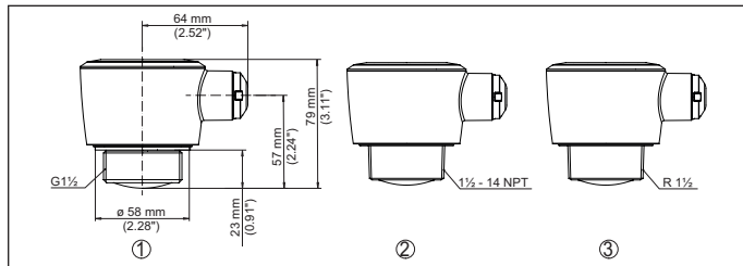
Abb. 22: Maße VEGAPULS C 22
