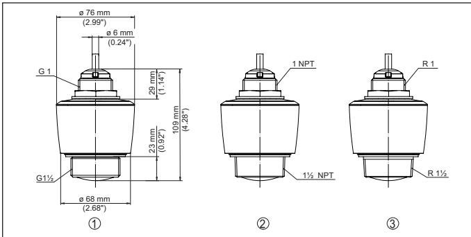
插图. 21: VEGAPULS C 11 尺寸
