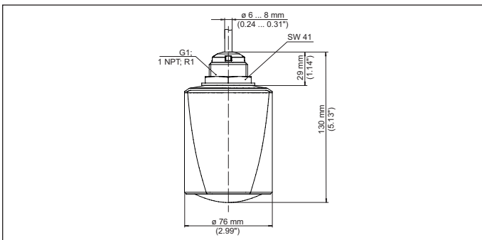
插图. 24: VEGAPULS C 23 尺寸
