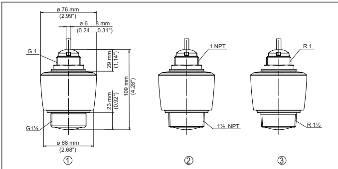
插图. 22: VEGAPULS C 21 尺寸
