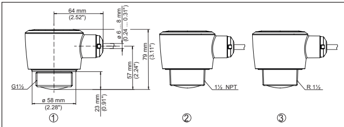
插图. 23: VEGAPULS C 22 尺寸
