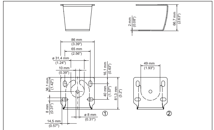
插图. 26: 用于天花板式安装的龙门框
