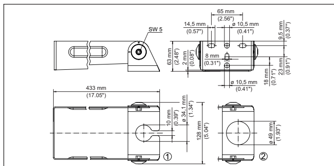
插图. 27: 安装到墙壁上时用的龙门框 - 悬臂 200 mm
