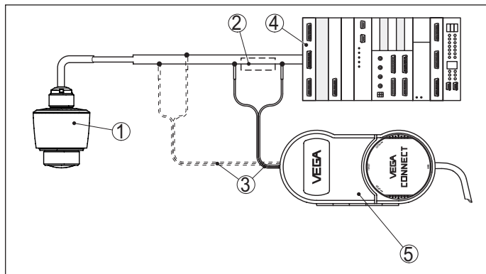
Fig. 19: Raccordement du PC à la ligne signal
