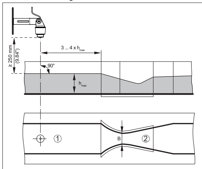
Fig. 11: Mesure du débit avec canal Venturi Khafagi : h_{\text{max}} = remplissage max. du canal ; B = resserrement max. du canal
