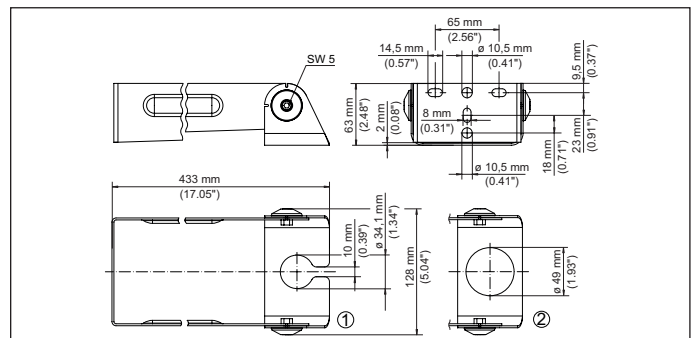
Fig. 26: Support de montage pour montage mural - potence 200 mm
