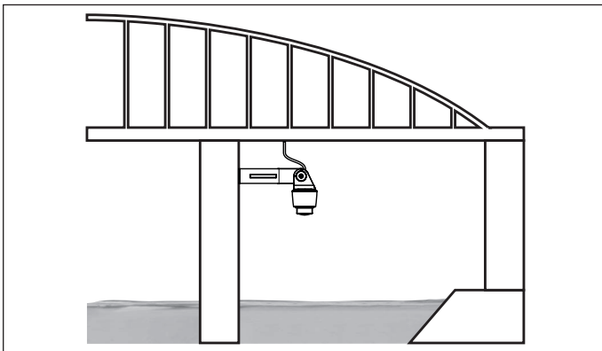
Fig. 8: Mesure de hauteur d'eau cours d'eau, Smontage du capteur sur un pilier de pont
