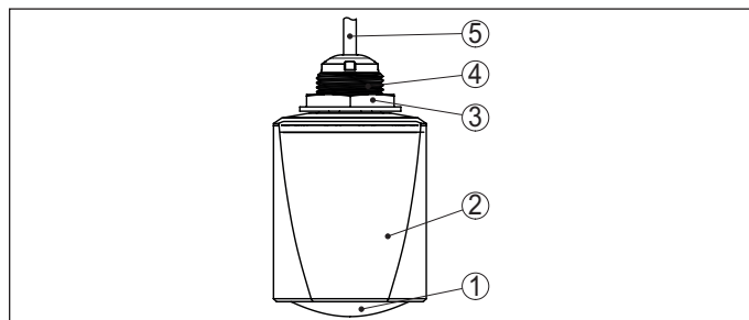
Fig. 4: VEGAPULS C 23 avec sortie de câble directe en protection IP66/IP68 (3 bar)
