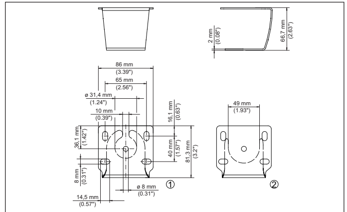
Fig. 25: Support de montage pour montage sur toit
