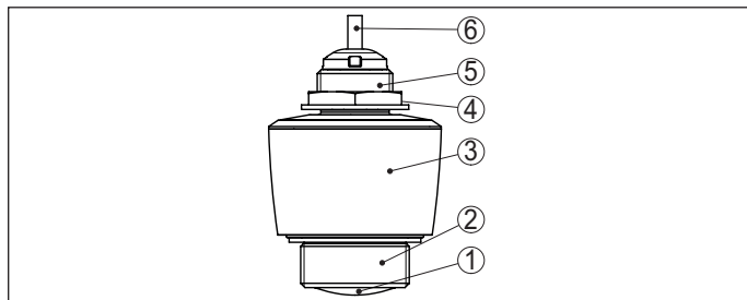
Fig. 2: VEGAPULS C 11 avec sortie de câble directe en protection IP66/IP68 (3 bar)
