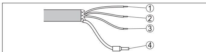
Fig. 16: Affectation des conducteurs du câble de raccordement raccordé de façon fixe
