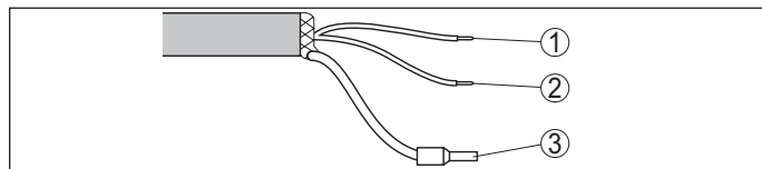
Fig. 14: Affectation des conducteurs du câble de raccordement raccordé de façon fixe
