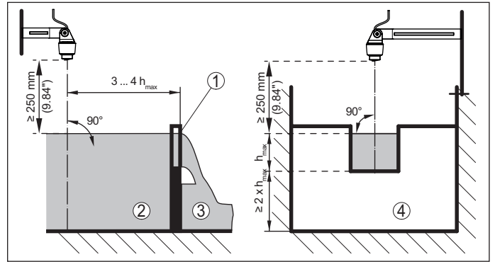
Fig. 10: Mesure du débit avec déversoir rectangulaire: h_{max} = remplissage max. du déversoir rectangulaire
