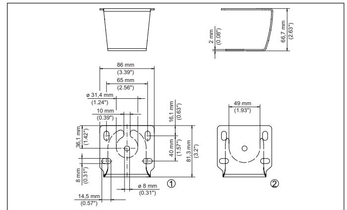
Fig. 26: Support de montage pour montage sur toit
