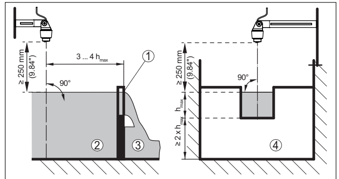
Figura 10: Misura di portata con stramazzo rettangolare: h_{max} = max. riempimento dello stramazzo rettangolare
