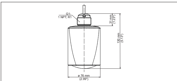
Figura 23: Dimensioni VEGAPULS C 23
