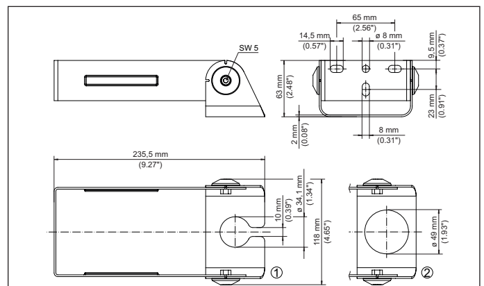
Figura 26: Staffa di montaggio per il montaggio a parete - braccio di supporto 200 mm
