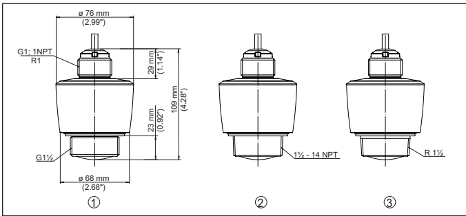
Figura 21: Dimensioni VEGAPULS C 11, C 21
