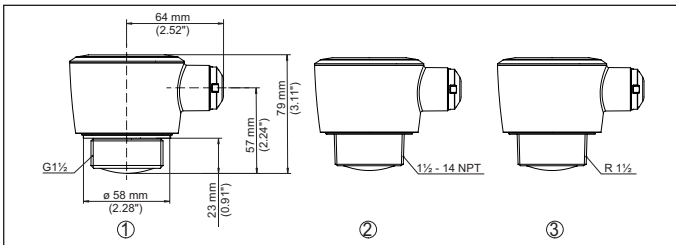
Figura 22: Dimensioni VEGAPULS C 22
