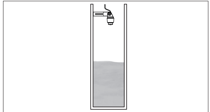
Figura 9: Misura d'altezza pozzo profondo, montaggio del sensore sul coperchio
