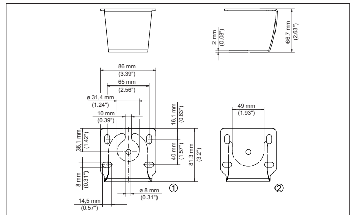
Figura 25: Staffa di montaggio per montaggio a soffitto
