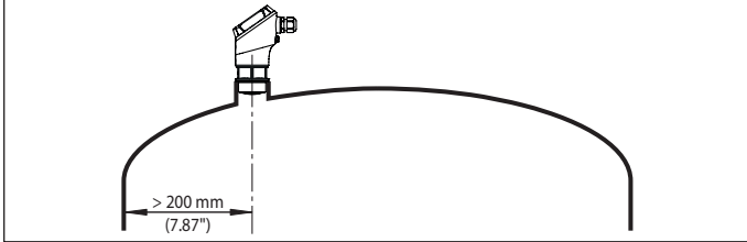
Fig. 6: Montage van de radarsensor op ronde tankdaken
