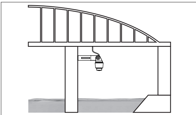
Fig. 8: Peilmeting rivier, sensormontage op brugpijler
