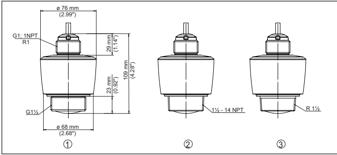
Fig. 21: Afmetingen VEGAPULS C 11, C 21
