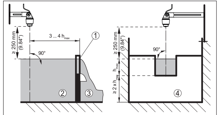
Fig. 10: Flowmeting met rechthoekig overstortschot: h_{max} = max. vulling van het rechthoekig overstortschot
