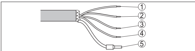
Fig. 17: Aderbezetting vast aangesloten aansluitkabel
