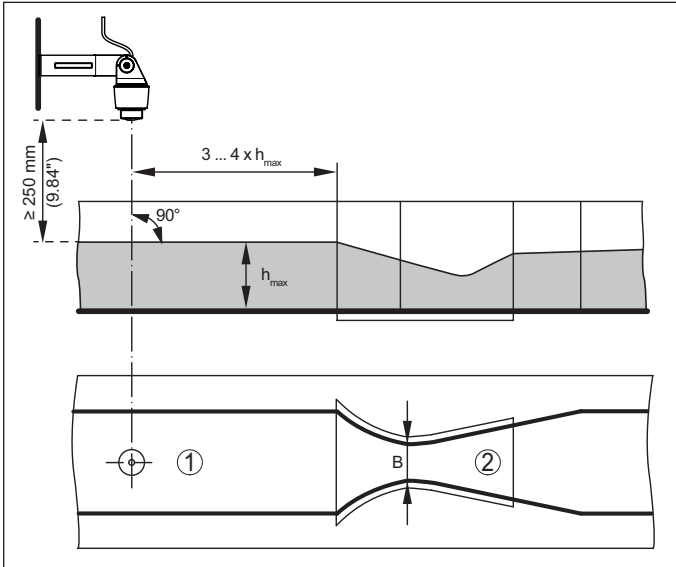
Fig. 11: Flowmeting met Khafagi-venturigoot: h_{max} = max. peil in de goot; B = maximale insnoering van de goot
