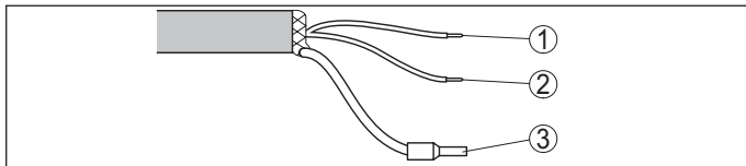
Fig. 14: Aderbezetting vast aangesloten aansluitkabel
