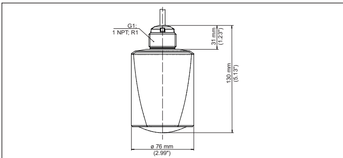
Fig. 23: Afmetingen VEGAPULS C 23
