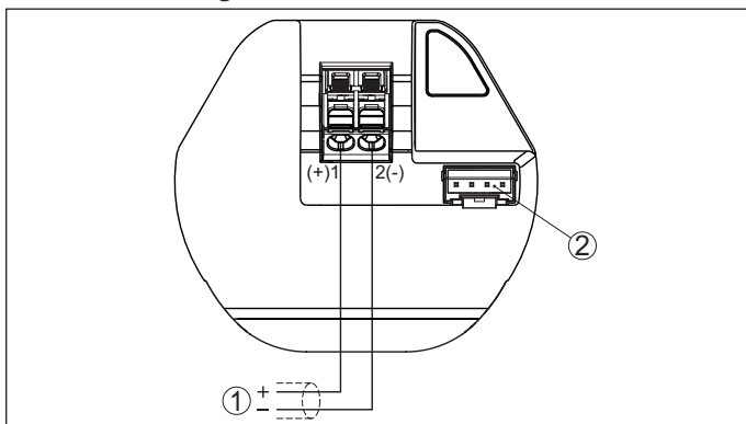
Fig. 15: Aansluitruimte VEGAPULS
