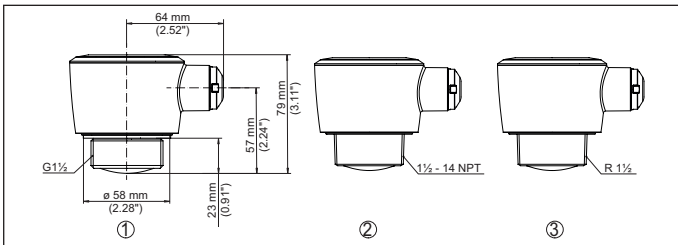
Fig. 22: Afmetingen VEGAPULS C 22
