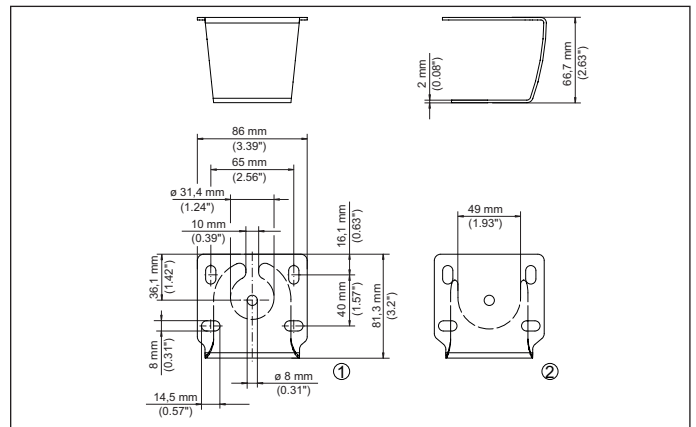
Fig. 25: Montagebeugel voor plafondmontage
