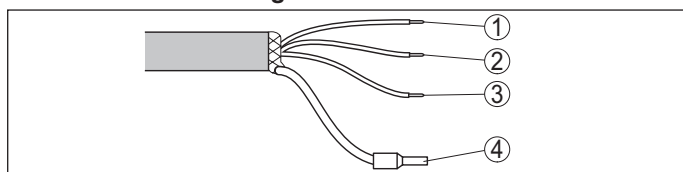
Fig. 16: Aderbezetting vast aangesloten aansluitkabel
