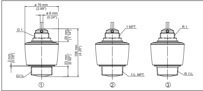
Fig. 21: Afmetingen VEGAPULS C 11
