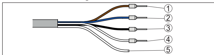
Fig. 17: Aderbezetting vast aangesloten aansluitkabel
