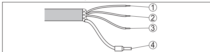
Fig. 16: Aderbezetting vast aangesloten aansluitkabel
