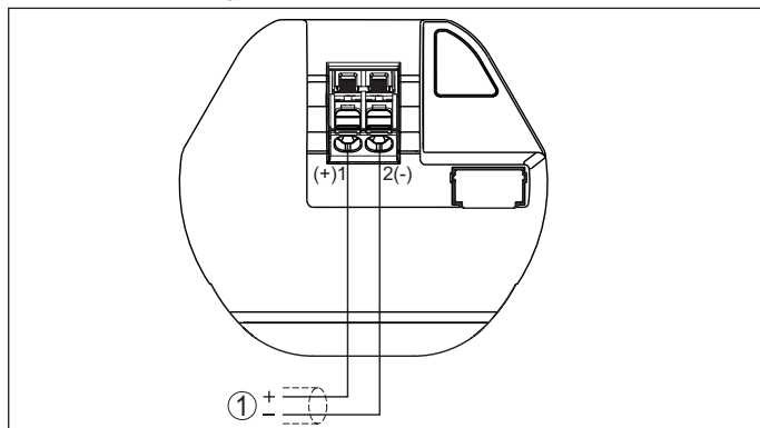
Fig. 13: Aansluitruimte VEGAPULS
