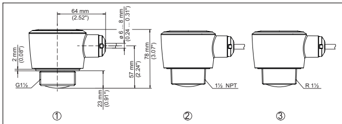
Fig. 23: Afmetingen VEGAPULS C 22
