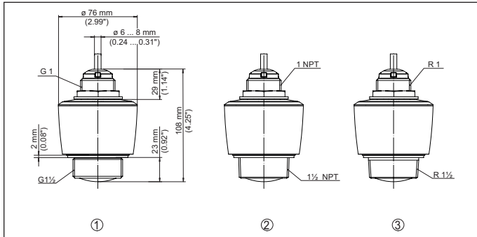
Fig. 22: Afmetingen VEGAPULS C 21
