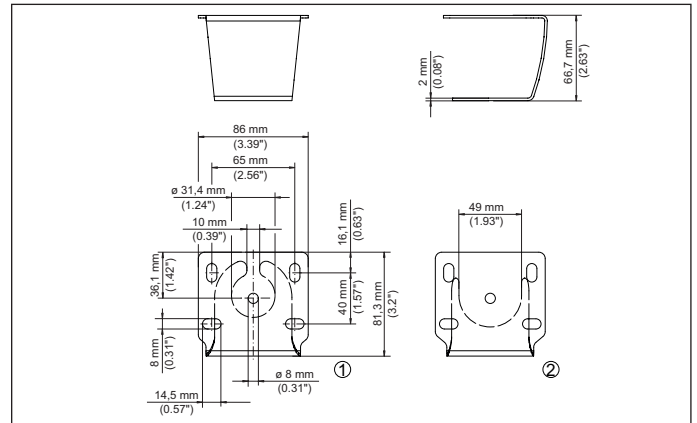
Fig. 26: Montagebeugel voor plafondmontage
