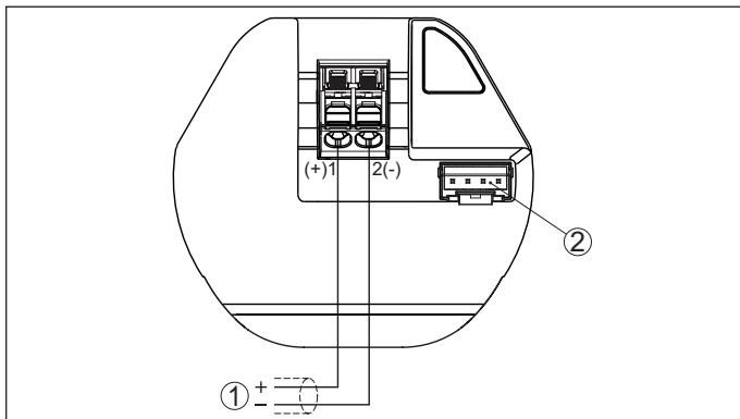
Fig. 15: Aansluitruimte VEGAPULS
