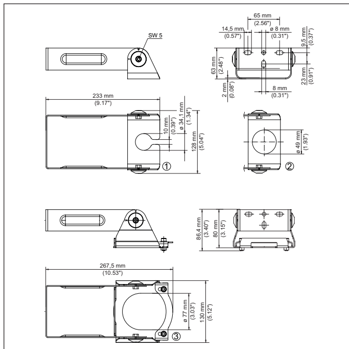
Fig. 27: Montagebeugel voor wandmontage - beugel 200 mm
