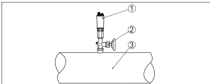
Abb. 10: Prozessdruckmessung von Gasen in Rohrleitungen
