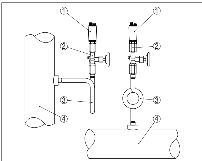
Abb. 11: Prozessdruckmessung von Dämpfen in Rohrleitungen
