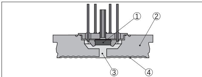
Abb. 2: Aufbau des Messsystems mit piezoresistivem Sensorelement
