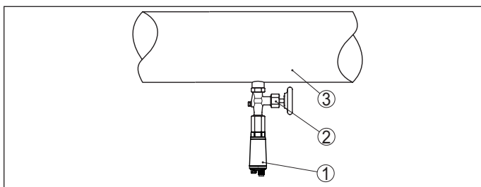
Abb. 12: Prozessdruckmessung von Flüssigkeiten in Rohrleitungen
