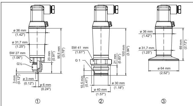
Abb. 24: Maße VEGABAR 28
