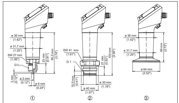
Figura 26: Dimensioni VEGABAR 38
