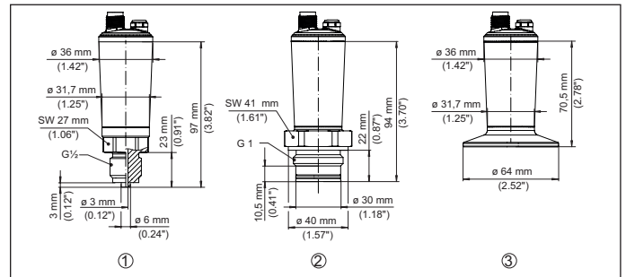
Figura 25: Dimensioni VEGABAR 29
