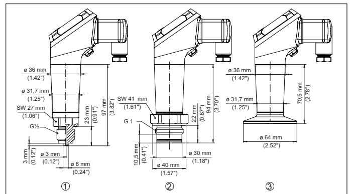
Figura 27: Dimensioni VEGABAR 39
