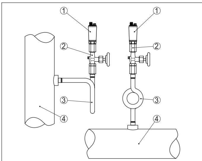
Fig. 11: Procesdrukmeting van stoom in leidingen
