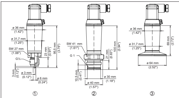
Fig. 24: Afmetingen VEGABAR 28
