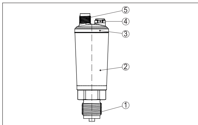
Fig. 7: VEGABAR 28 met M12 x 1-stekkerverbinding in beschermingsklasse IP66/IP67
