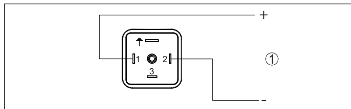
Fig. 14: Aansluitschema - tweedraads 4 ... 20 mA - stekker conform ISO 4400
