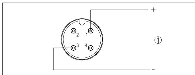
Fig. 13: Aansluitschema - tweedraads 4 ... 20 mA - M12 x 1-stekker
