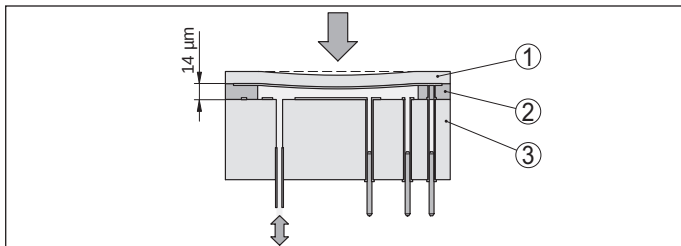
Fig. 1: Opbouw van de mini-CERTEC®-meetcel
