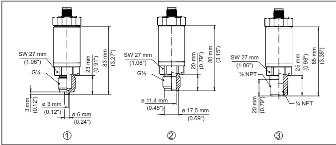
Fig. 22: Afmetingen VEGABAR 18
