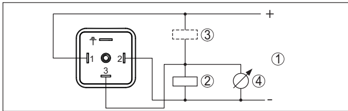
Fig. 18: Aansluitschema - driedraads (1 x transistor of 4 ... 20 mA)
