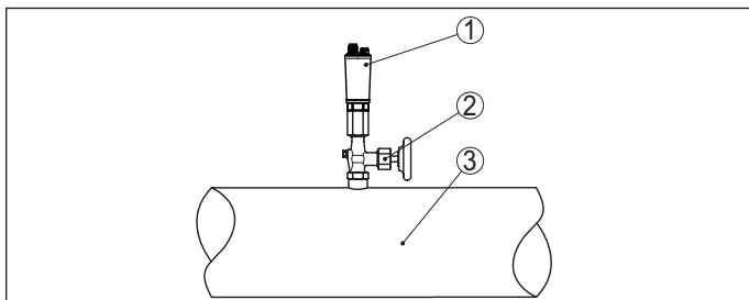
Fig. 10: Procesdrukmeting van gassen in leidingen
