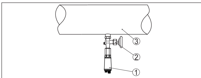
Fig. 12: Procesdrukmeting van vloeistoffen in leidingen
