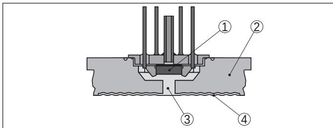
Fig. 2: Opbouw van het meetsysteem met piëzoresistief sensorelement
