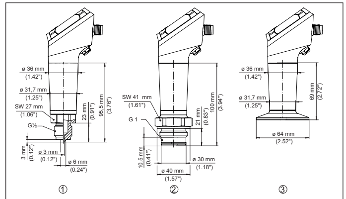
Fig. 26: Afmetingen VEGABAR 38
