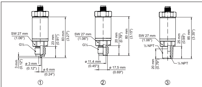
Fig. 23: Afmetingen VEGABAR 19
