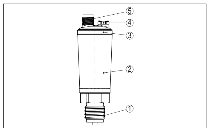
Fig. 7: VEGABAR 28 met M12 x 1-stekkerverbinding in beschermingsklasse IP66/IP67
