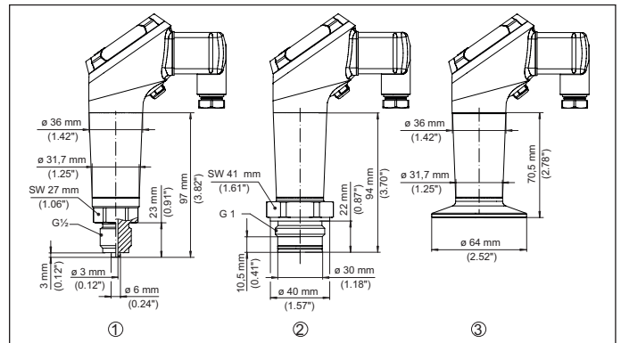
Fig. 27: Afmetingen VEGABAR 39
