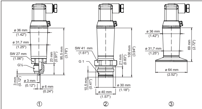
Fig. 24: Afmetingen VEGABAR 28
