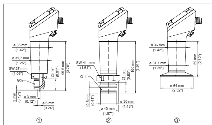
Rys. 26: Wymiary VEGABAR 38
