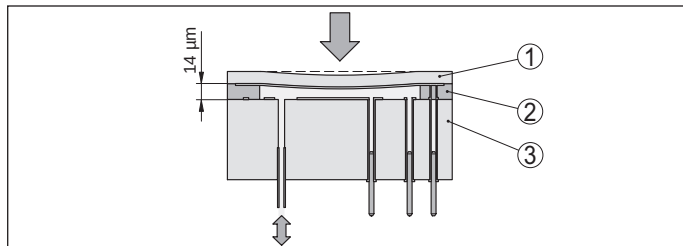
Rys. 1: Budowa komórki pomiarowej Mini-CERTEC®
