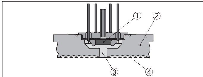
Rys. 2: Budowa układu pomiarowego z czujnikami piezorezystancyjnym
