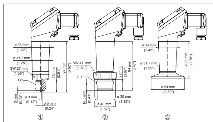
Rys. 27: Wymiary VEGABAR 39
