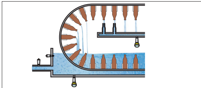
Fig. 2: Detección de nivel en sistema de limpieza de botellas
