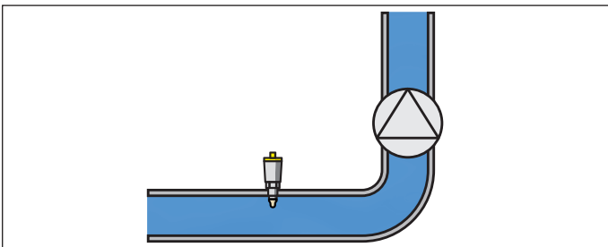
Fig. 5: Protección contra marcha en seco en tuberías
