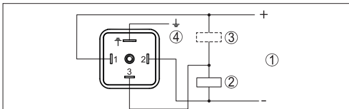
Fig. 11: Esquema de conexión enchufe ISO 4400 - salida de transistor de tres hilos
