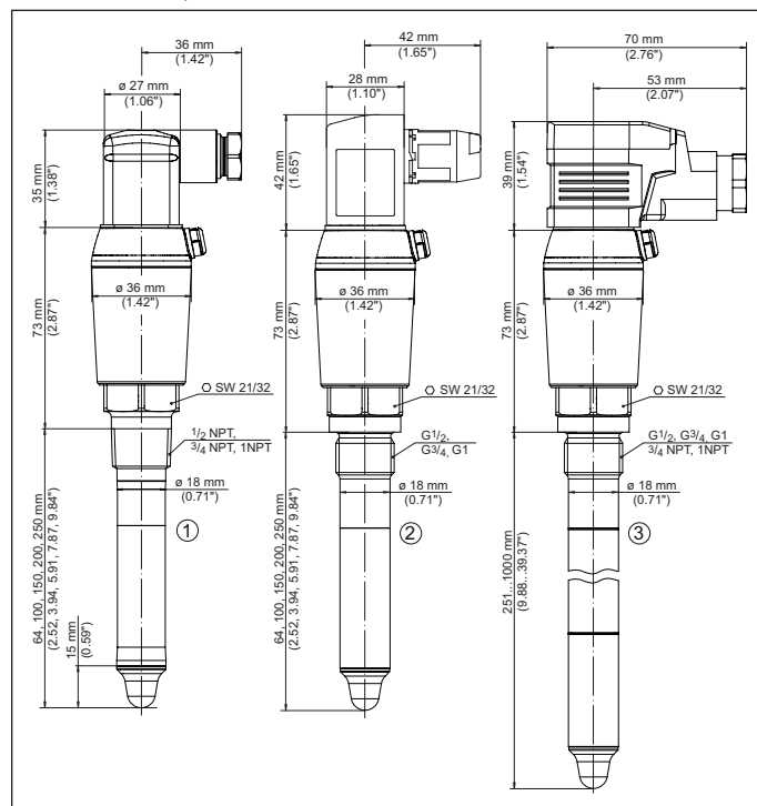
Fig. 18: VEGAPOINT, Versión estándar - Rosca, con enchufe para válvula según ISO 4400
