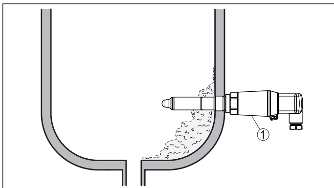
Fig. 10: Montaje lateral - Depósitos
