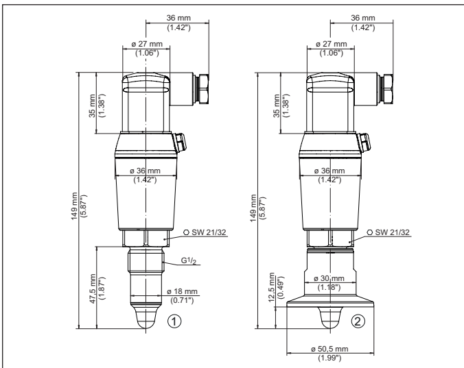
Fig. 20: VEGAPOINT, versión higiénica - rosca, con enchufe ISO 4400
