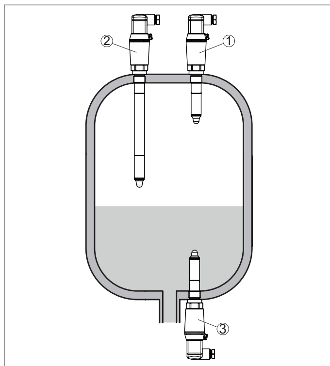
Fig. 7: Ejemplos de instalación - VEGAPOINT 23
