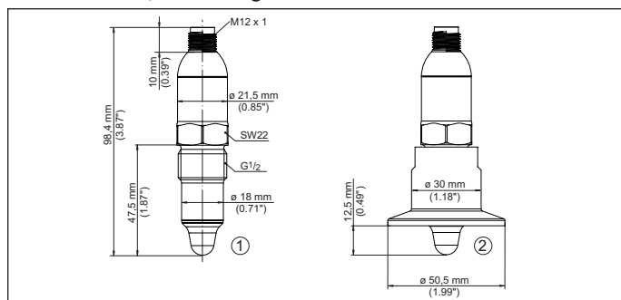
Fig. 15: VEGAPOINT, versión higiénica - Rosca
