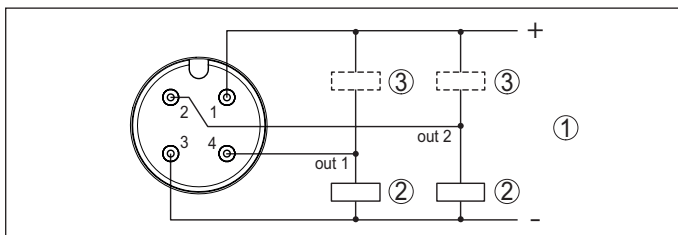
Fig. 12: Esquema de conexiones conector M12 x 1 - Salida de transistor, tres hilos.
