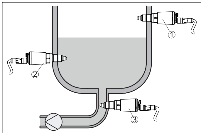
Fig. 6: Ejemplos de instalación - VEGAPOINT 21
