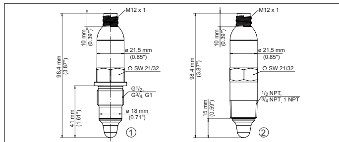
Fig. 14: VEGAPOINT, versión estándar - rosca
