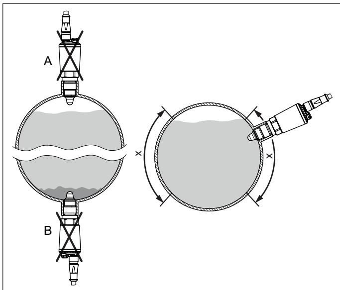
Fig. 9: Montaje en tuberías horizontales
