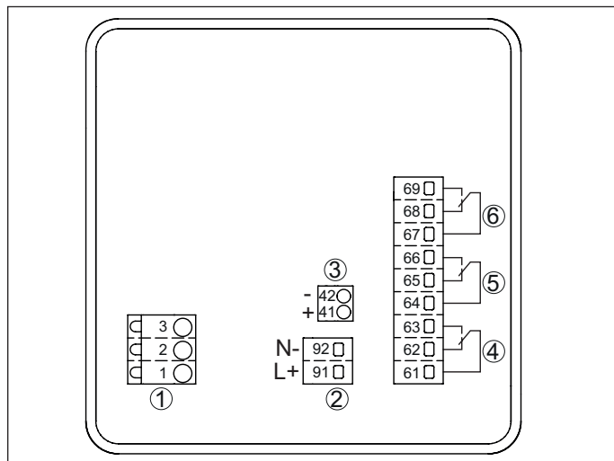
插图. 9: VEGAMET 341 的接线图
