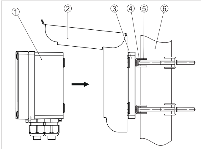
插图. 6: 将遮阳罩安装在管件上
