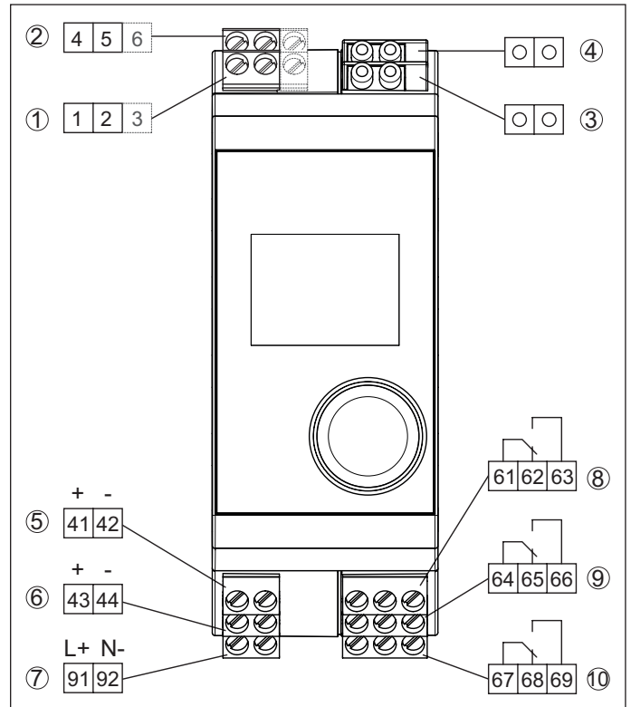
插图. 8: VEGAMET 142 的接线图
