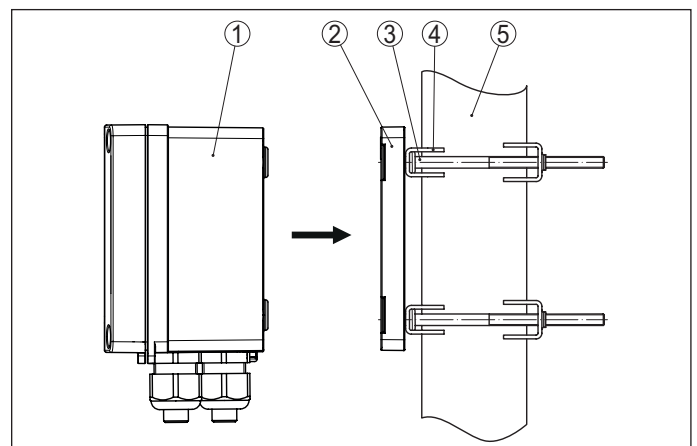
插图 5: 管式安装
