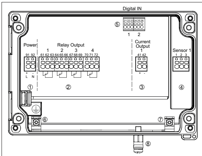
插图. 13: VEGAMET 的接线图
