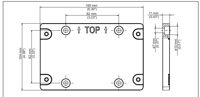
插图. 21: VEGAMET 841, 842 安装板的尺寸
