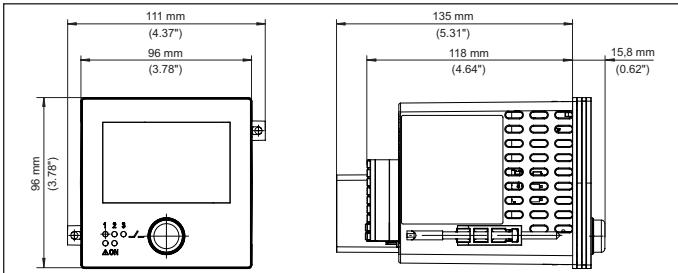
插图. 18: VEGAMET 341 的尺寸
