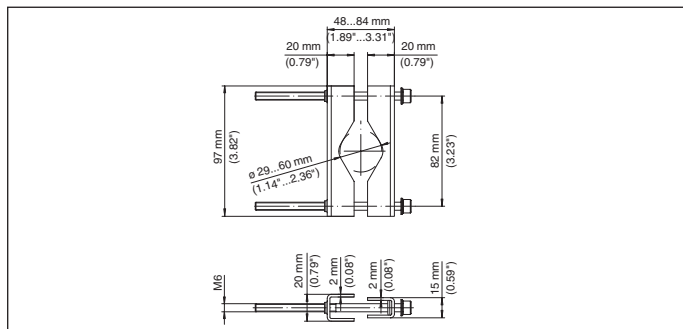
插图. 27: VEGAMET 861, 862 管件式安装用夹子的尺寸
