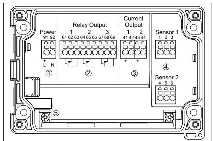
插图. 12: VEGAMET 的接线图
