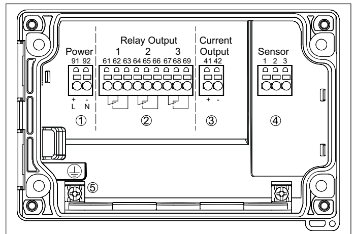
插图. 11: VEGAMET 的接线图
