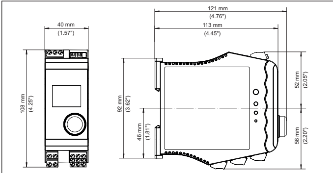
插图. 16: VEGAMET 141 的尺寸
