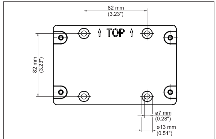
插图 3: 壁挂式安装用的安装板 (VEGAMET 841, 842)
