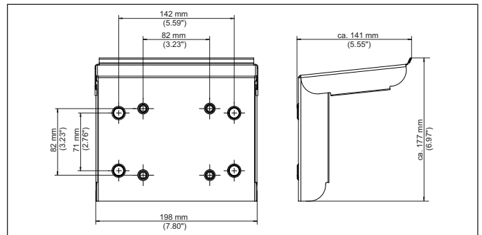
插图. 22: VEGAMET 841, 842 遮阳罩的尺寸
