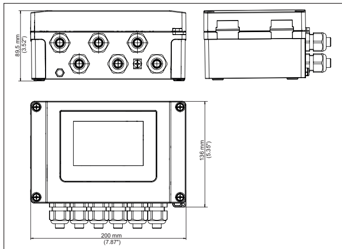
插图. 24: VEGAMET 861, 862 的尺寸
