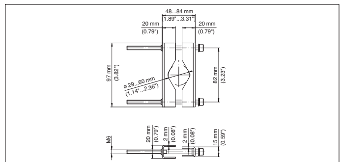
插图. 23: VEGAMET 841, 842 管件式安装用夹子的尺寸
