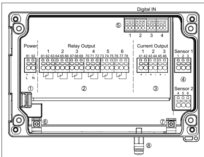
插图. 14: VEGAMET 的接线图
