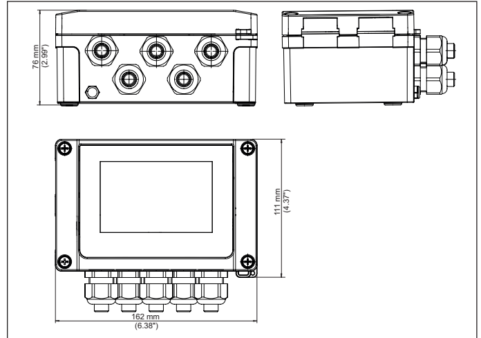
插图. 20: VEGAMET 841, 842 的尺寸
