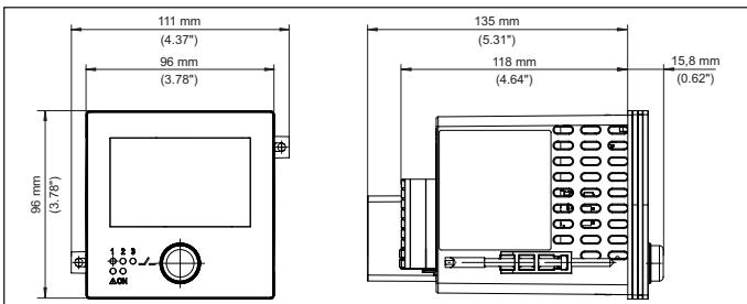
插图. 19: VEGAMET 342 的尺寸
