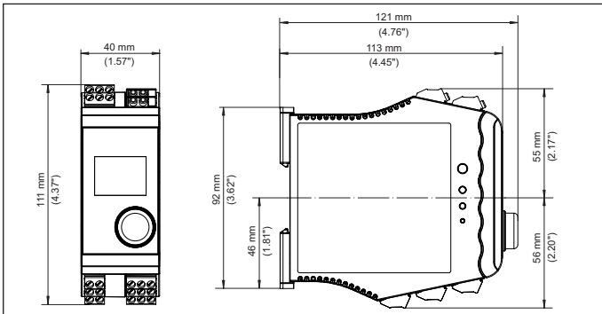
插图. 17: VEGAMET 142 的尺寸
