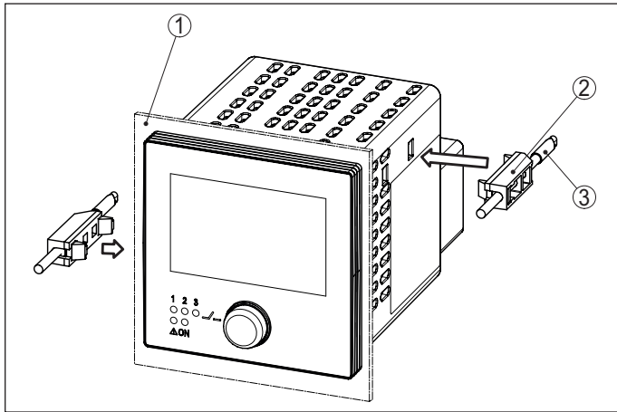
插图 2: 安装在控制面板内
