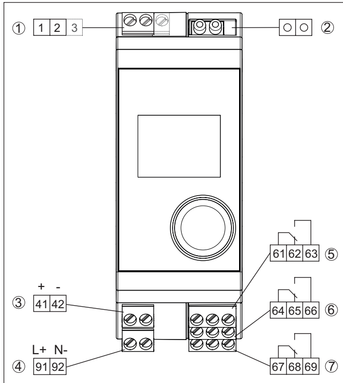
插图. 7: VEGAMET 141 的接线图
