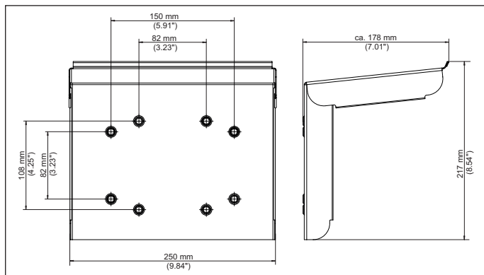
插图. 26: VEGAMET 861, 862 遮阳罩的尺寸
