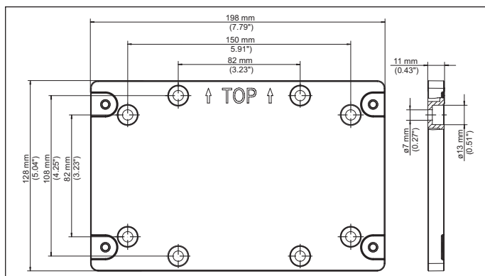
插图. 25: VEGAMET 861, 862 安装板的尺寸
