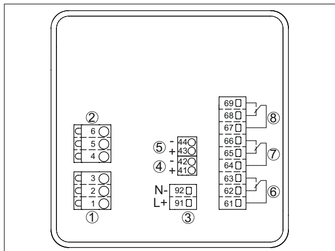
插图. 10: VEGAMET 342 的接线图
