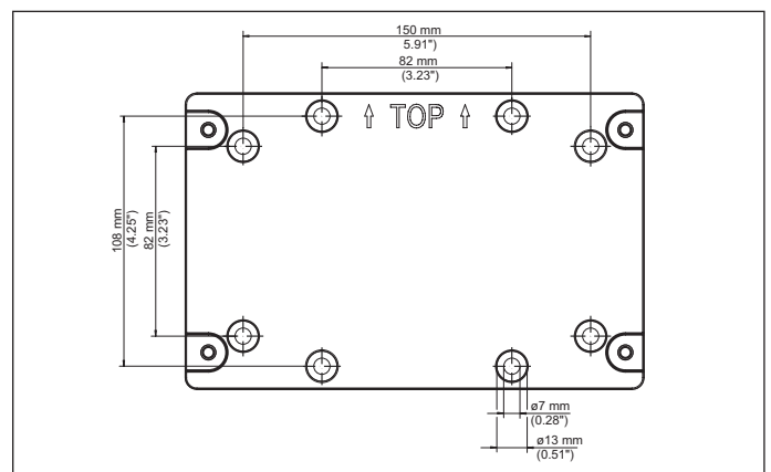
插图 4: 壁挂式安装用的安装板 (VEGAMET 861, 862)
