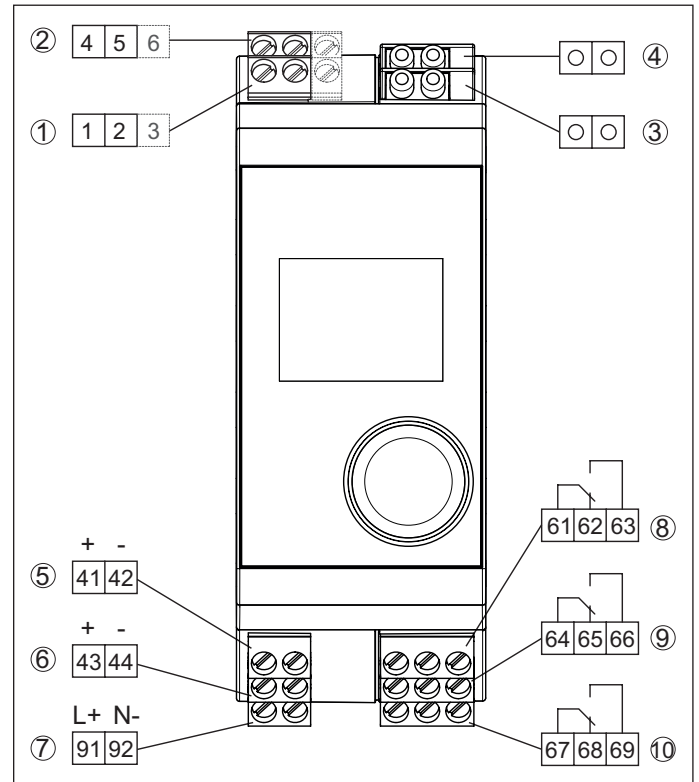
Fig. 8: Wiring plan VEGAMET 142
