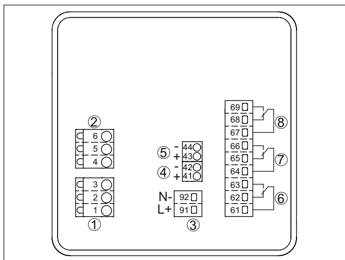
Figura 10: Schema di collegamento VEGAMET 342
