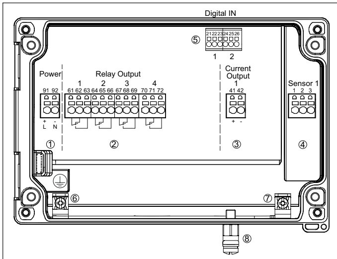
Figura 13: Schema di allacciamento VEGAMET
