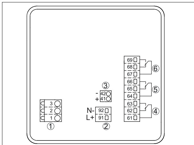
Figura 9: Schema di collegamento VEGAMET 341
