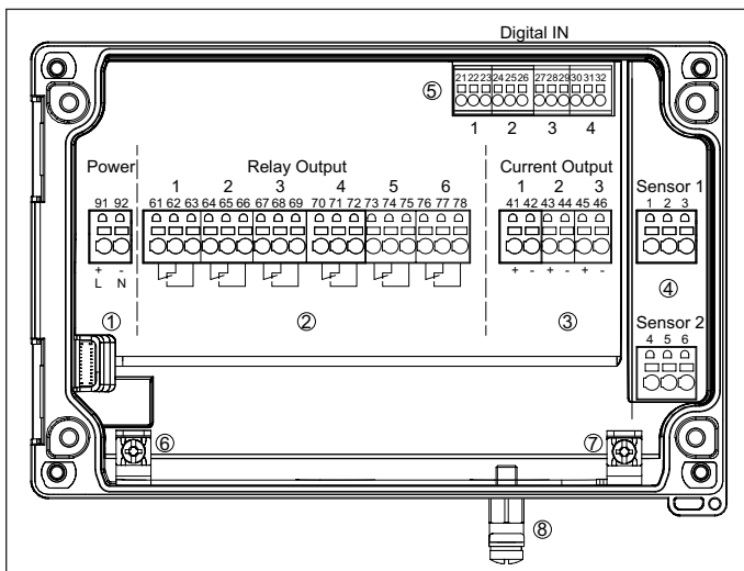
Figura 14: Schema di allacciamento VEGAMET
