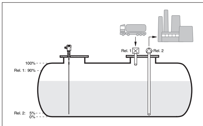
Figura 16: Esempio di misura di livello in un serbatoio cilindrico orizzontale
