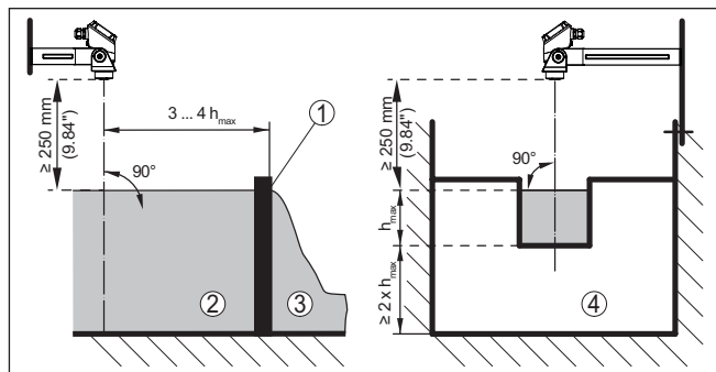
Figura 24: Misura di portata con stramazzo rettangolare: h_{max} = \text{max. riempimento dello stramazzo rettangolare}
