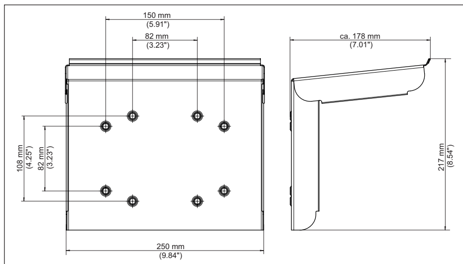
Fig. 28: Afmetingen zonnedak
