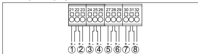
Fig. 9: Aansluiting van de digitale ingangen
