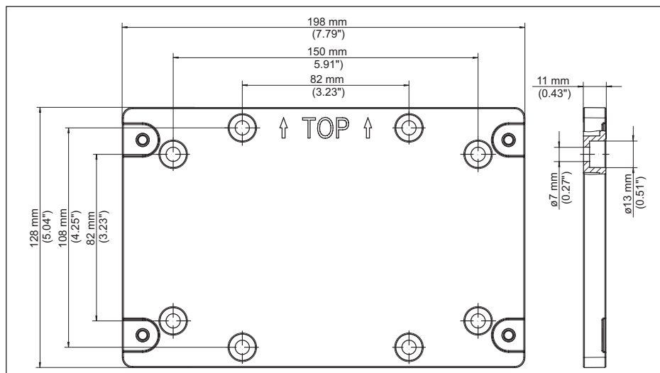
Fig. 27: Afmetingen montageplaat
