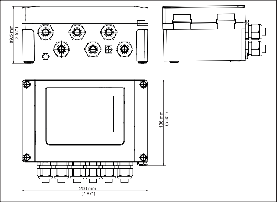
Fig. 26: Afmetingen VEGAMET 862
