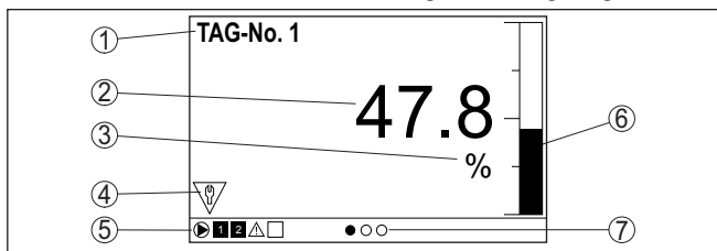
Fig. 12: Voorbeeld meetwaarde-indicatie (meetwaarde met bargraph)
