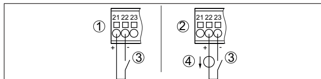
Fig. 10: Asignación de conexión de las entradas digitales (activo/pasivo)
