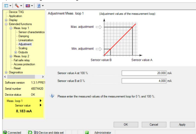
Fig. 15: Ejemplo de una vista DTM - Ajuste
