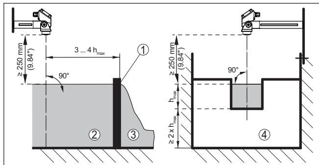
Fig. 24: Medición de caudal con canal rectangular: h_{\max} = llenado máx. del canal rectangular
