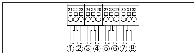
Fig. 9: Conexión de las entradas digitales
