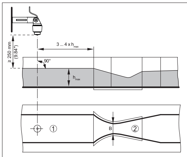
Fig. 25: Medición de caudal con canal venturi Khafagi: h_{\max} = llenado máx. del canal; B = mayor estrechamiento del canal
