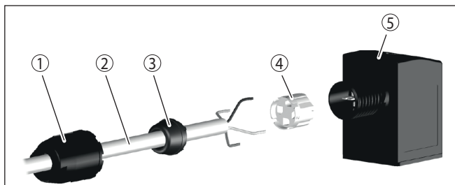
Abb. 9: Anschluss Ventilstecker ISO 4400 mit Schneidklemmtechnik
