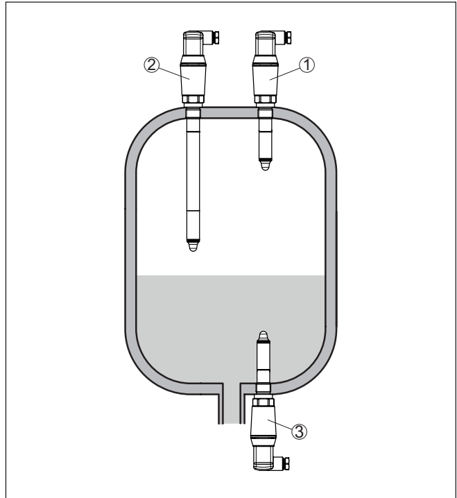
Abb. 4: Einbaubeispiele
