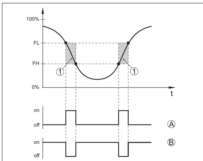
Abb. 14: Fensterfunktion
