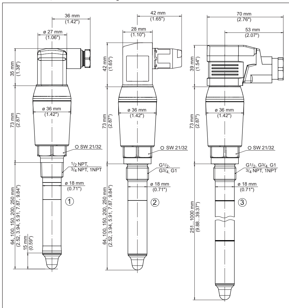
Abb. 20: VEGAPOINT 23, Standardausführung - Gewinde, mit Ventilsteckern nach ISO 4400
