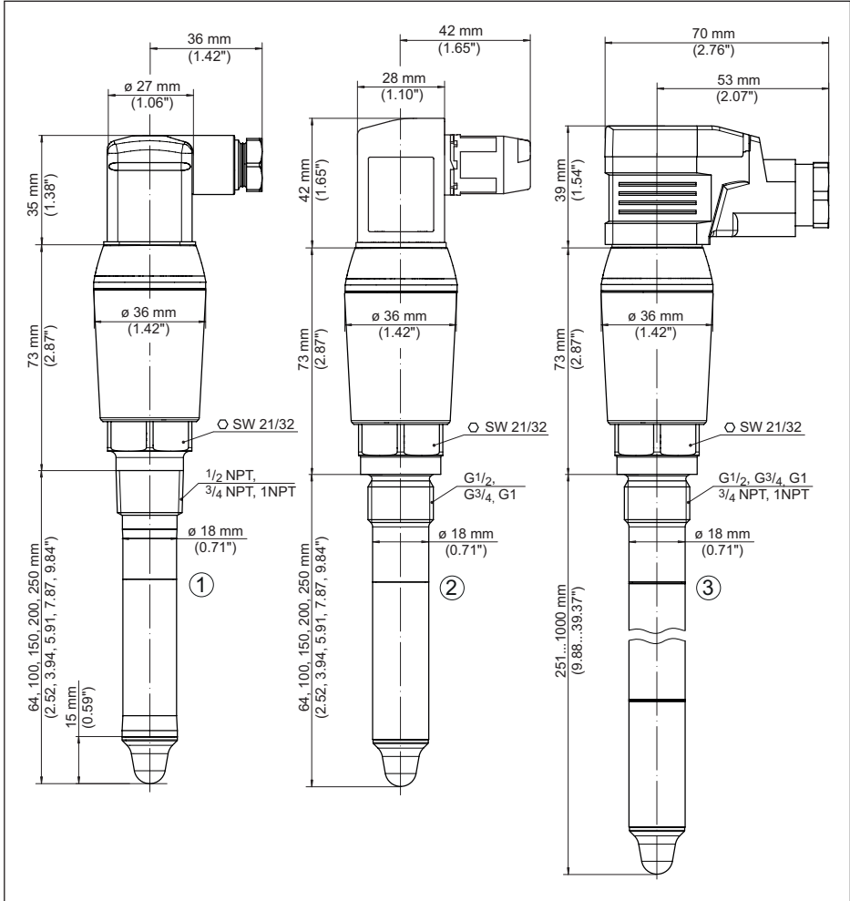
Res. 20: VEGAPOINT 23, Standart model - dişli, ISO 4400'e uygun ventil fişli
