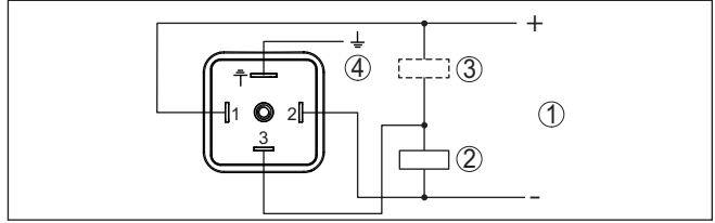
Res. 12: Bağlantı planı fiş ISO 4400 - Transistör çıkışı uç telli
