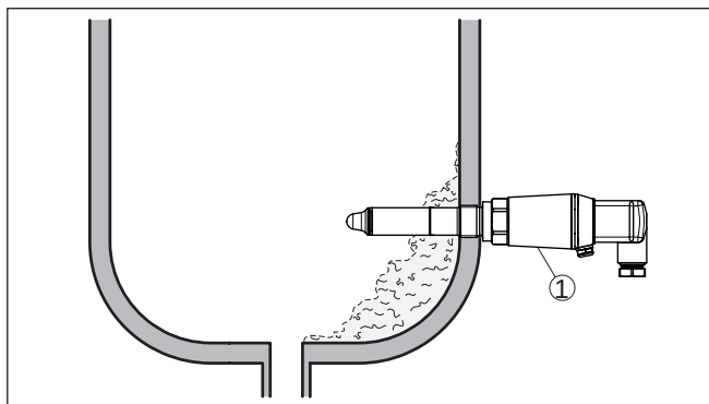
Fig. 5: Zijmontage - afzettingen
