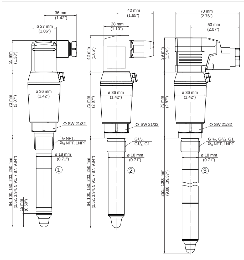
Fig. 19: VEGAPOINT 23, standaarduitvoering - schroefdraad, met ventielstekkers conform ISO 4400
