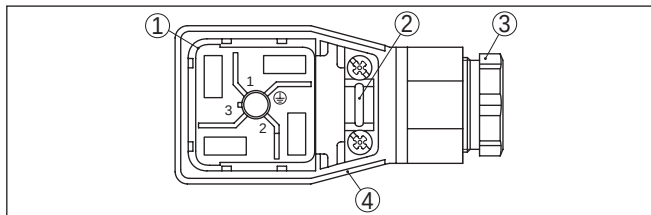
Fig. 9: Losmaken van het binnenwerk.
