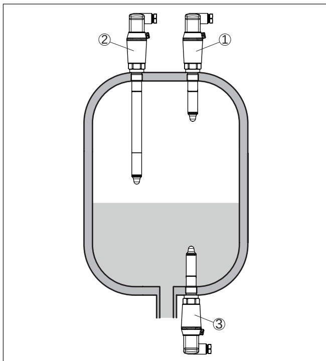
Fig. 4: Inbouwvoorbeelden
