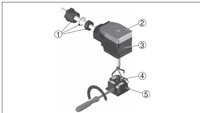
Fig. 10: Aansluiting op de schroefklemmen
