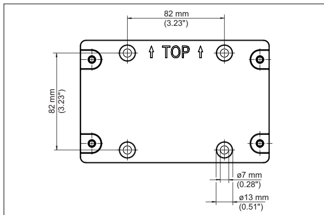
Figura 3: Piastra per montaggio a parete VEGAMET 842
