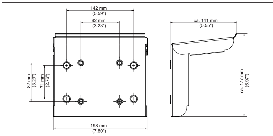
Fig. 26: Afmetingen zonnedak
