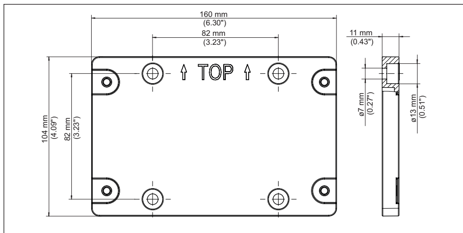
Fig. 25: Afmetingen montageplaat
