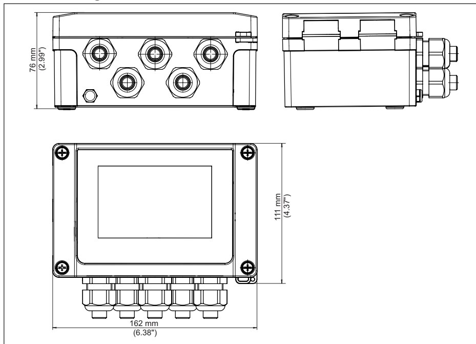
Fig. 24: Afmetingen VEGAMET 842
