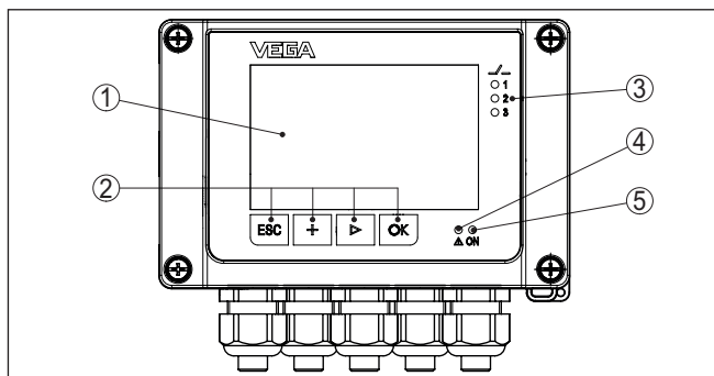
Fig. 9: Aanwijs- en bedieningselementen
