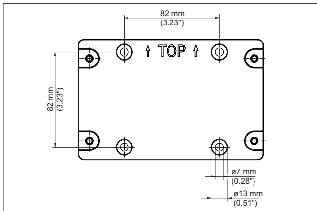
Fig. 3: Montageplaat voor wandmontage VEGAMET 842
