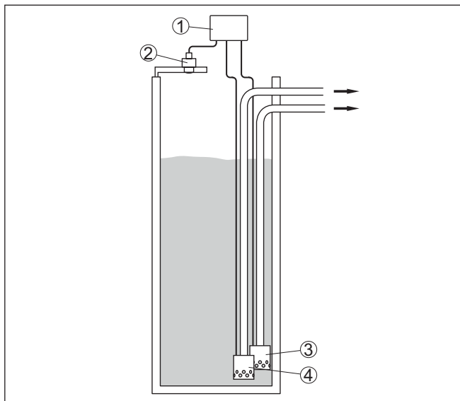
Fig. 15: Voorbeeld pompstation: pompregeling in inlaatschacht
