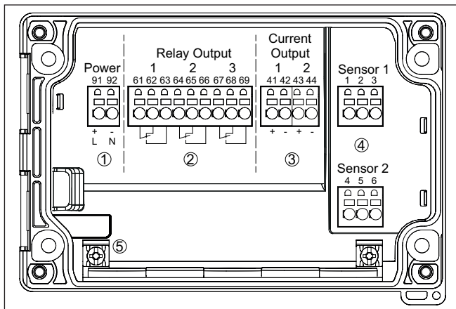
Fig. 6: Aansluitschema VEGAMET 842
