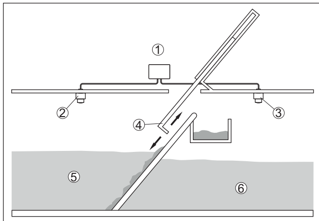
Fig. 21: Voorbeeld van een kroosrekbesturing
