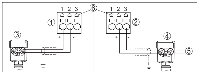
Fig. 7: Entrada conexión 1 para el sensor de dos/cuatro hilos (activo/pasivo)
