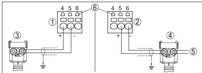
Fig. 8: Entrada conexión 2 para el sensor de dos/cuatro hilos (activo/pasivo)
