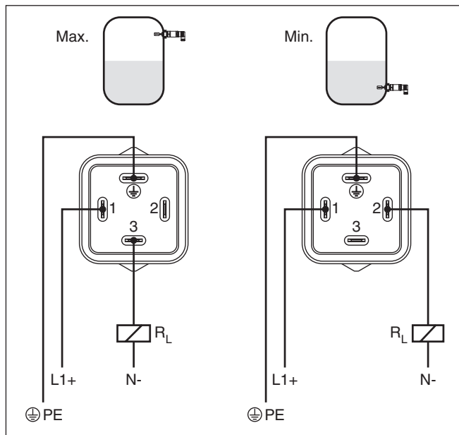
Fig. 13: Aansluitschema, contactloze schakelaar bij ventielconnector ISO 4400
