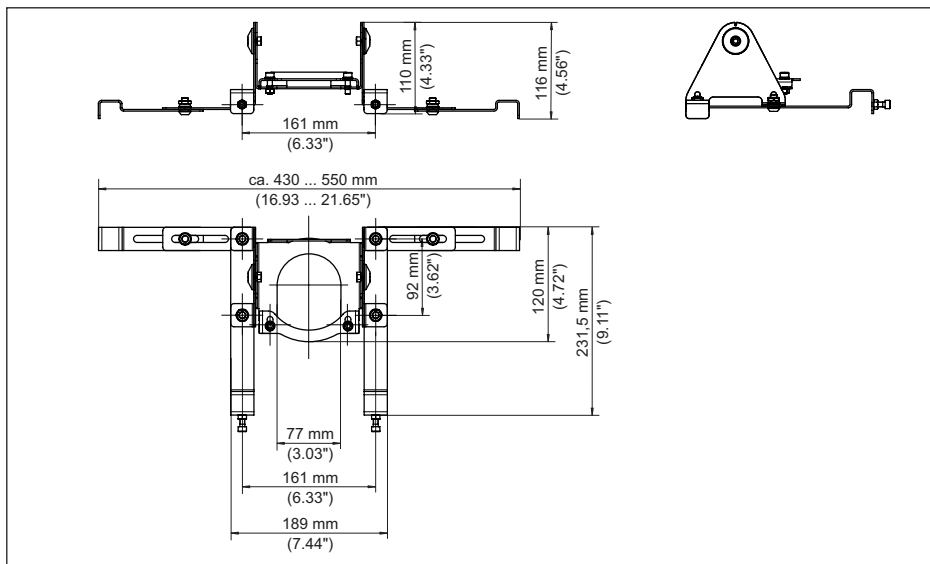
Fig. 30: Montagebeugel voor kunststof tank - met bevestiging voor IBC-container, sensorhouder 1½"
