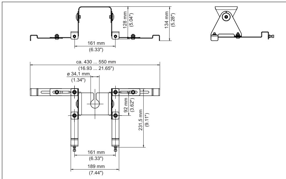
Fig. 29: Montagebeugel voor kunststof tank - met bevestiging voor IBC-container, sensorhouder 1"
