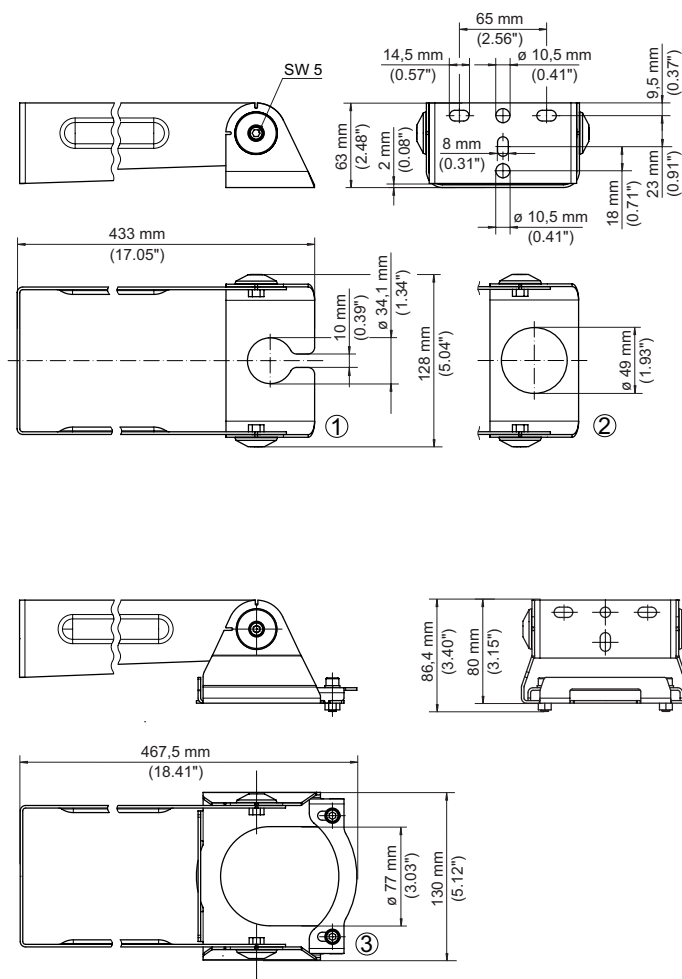
Fig. 24: Montagebeugel voor wandmontage, sensorhouder verstelbaar - beugel 400 mm
