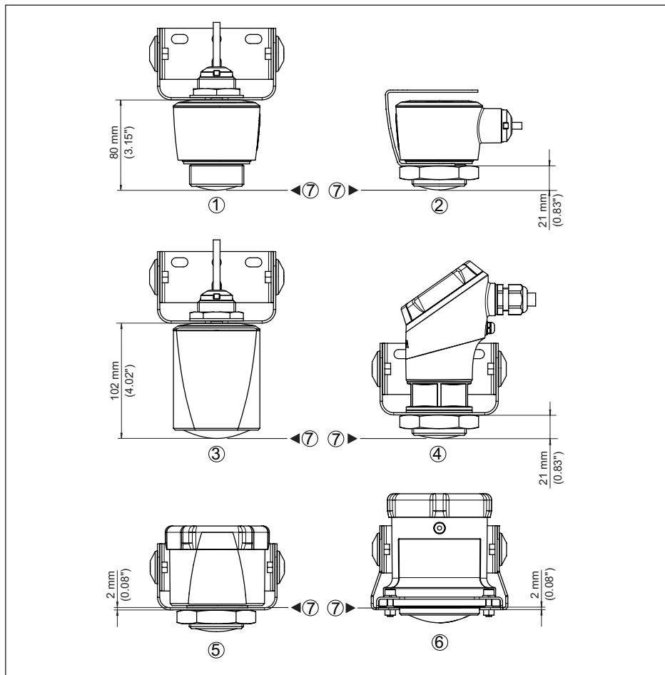
Fig. 32: Montagebeugel voor dak- en wandmontage - afstand van het sensorreferentievlak tot de onderkant van de sensorhouder.
