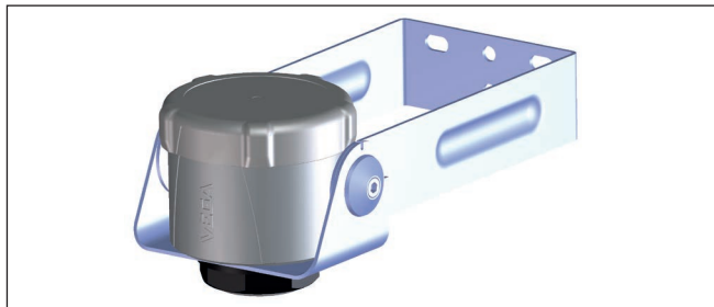
Fig. 11: Montagebeugel met verstelbare sensorhouder
