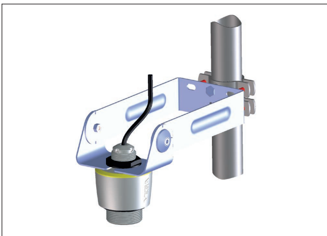
Fig. 17: Montagebeugel voor pijpmontage verticaal via buisklemmen
