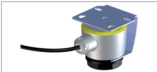
Fig. 9: Montagebeugel voor plafondmontage - sensorhouder voor G1½
