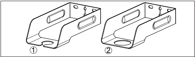
Fig. 3: Montagebeugel voor wandmontage - met vaste sensorhouder
