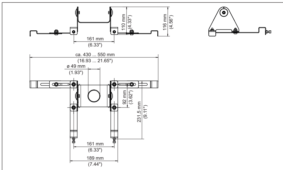
Fig. 31: Montagebeugel voor kunststof tank - met bevestiging voor IBC-container, sensorhouder voor overschuifflens
