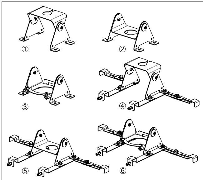
Fig. 6: Montagebeugel voor kunststof tanks - met verstelbare sensorhouder
