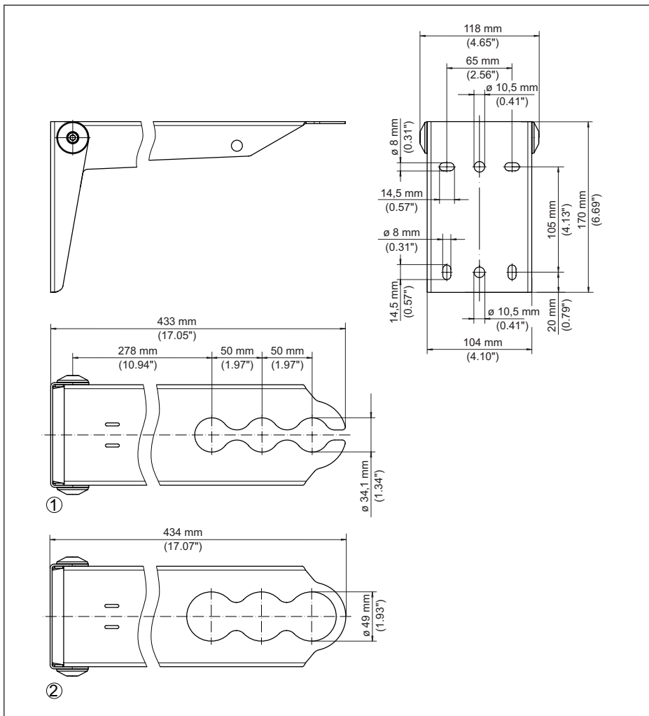
Fig. 26: Montagebeugel voor wandmontage, klapbaar
