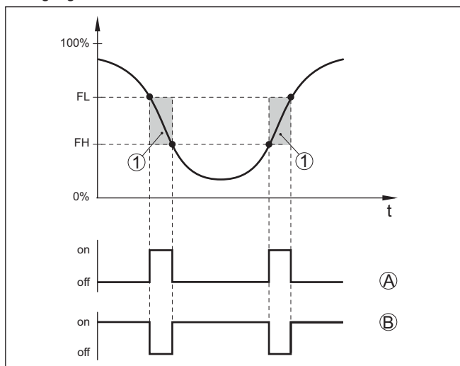
Fig. 9: Vensterfunctie
