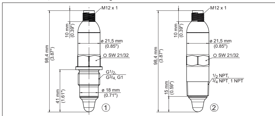
Fig. 11: VEGAPOINT 11, standaarduitvoering - schroefdraad
