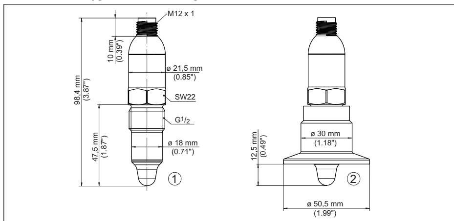
Fig. 12: VEGAPOINT 11, hygiënische uitvoering - schroefdraad
