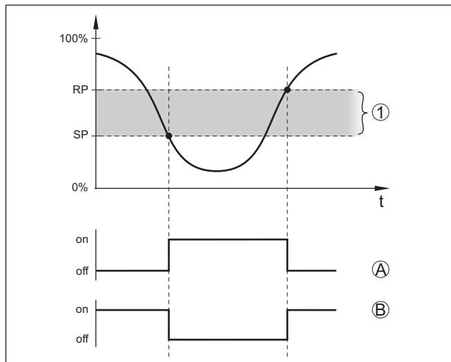
Fig. 8: Hysteresefunctie
