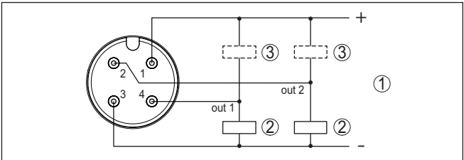
Fig. 7: Aansluitschema M12x1-stekker - transistoruitgang, driedraads
