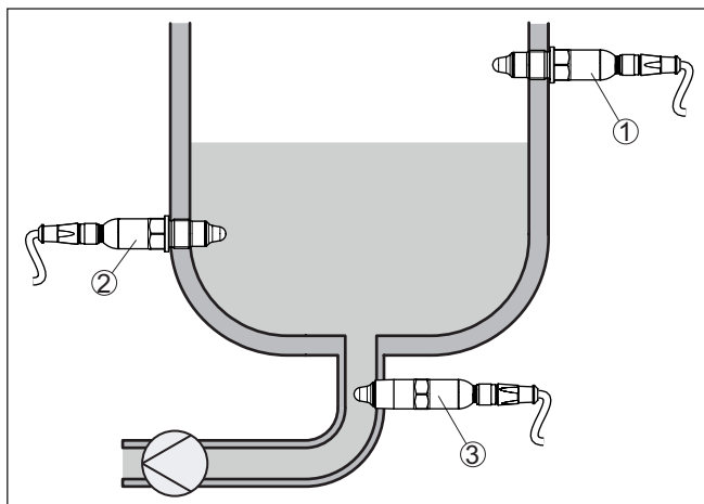
Fig. 3: Inbouwvoorbeelden
