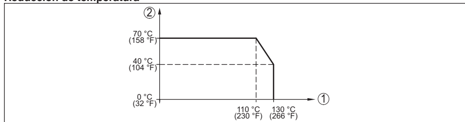
Abb. 4: Reducción de temperatura VEGABAR 28, 29
