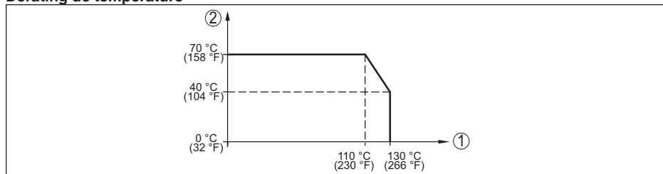
Abb. 3: Derating de température VEGABAR 28, 29
