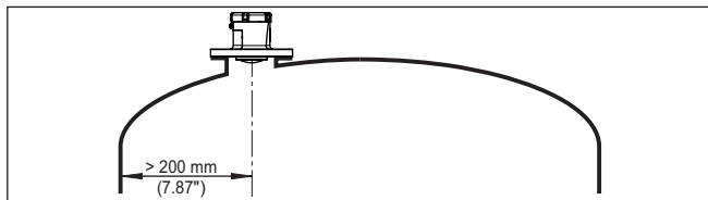
Fig. 5: Montage van de radarsensor op ronde tankdaken
