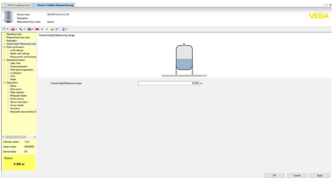
Fig. 23: Voorbeeld van een DTM-aanzicht - menupunt tankhoogte, meetbereik
