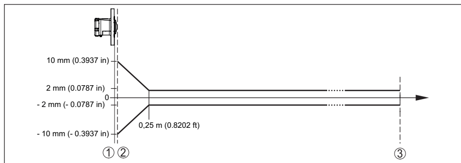
Fig. 28: Meetnauwkeurigheid onder referentiecondities
