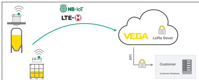
Fig. 17: Draadloze meetwaardeoverdracht via NB-IoT en LTE-M naar de VEGA cloud
