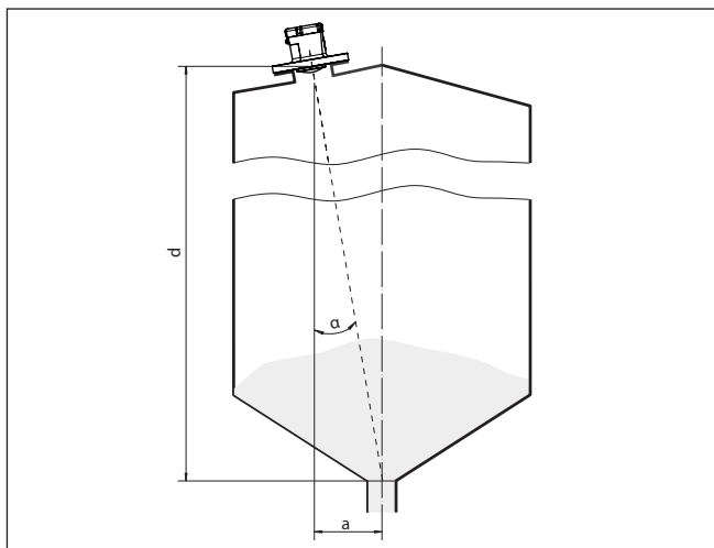
Fig. 12: Voorstel voor de inbouw na uitrichting VEGAPULS Air 42
