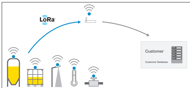
Fig. 18: Draadloze meetwaardeoverdracht
