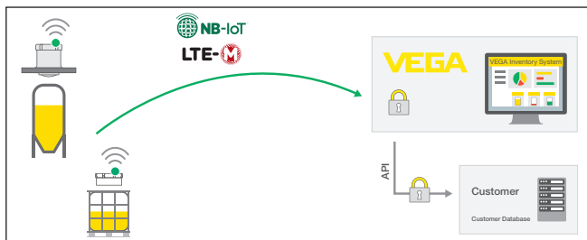
Fig. 15: Draadloze meetwaardeoverdracht via NB-IoT en LTE-M voor het VEGA Inventory System
