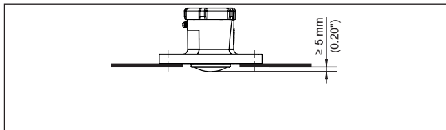
Fig. 8: Aanbevolen montage sok van de VEGAPULS Air 42
