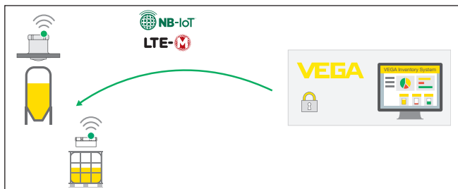
Fig. 25: Toegang op afstand vanuit het VEGA Inventory System via NB-IoT of LTE-M naar de sensor
