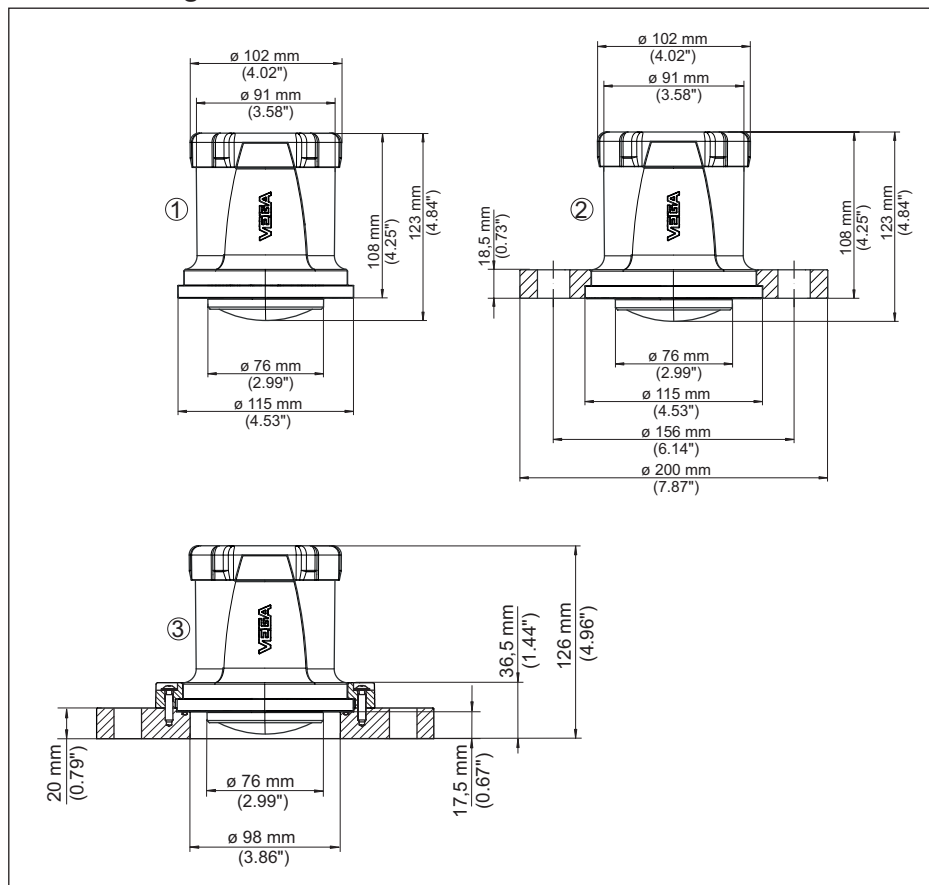
Fig. 29: Afmetingen VEGAPULS Air 42
