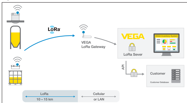
Fig. 16: Draadloze meetwaardeoverdracht via LoRaWAN, LoRa-server naar het VEGA Inventory System
