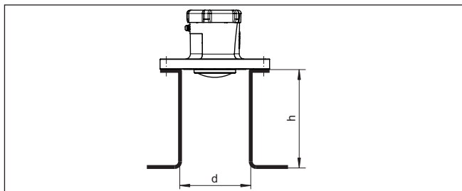
Fig. 9: Sokmontage bij afwijkende afmetingen
