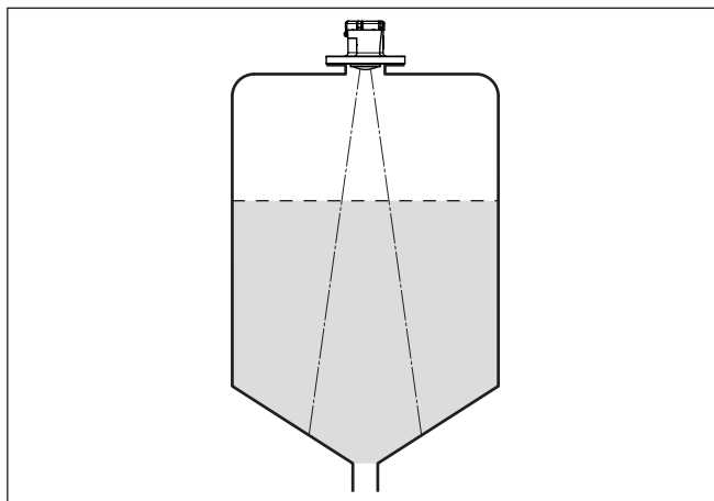
Fig. 6: Montage van de radarsensor op tanks met conische bodem
