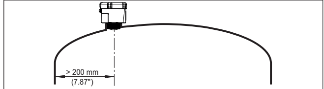
Fig. 5: Montage du capteur radar dans une cuve à toit bombé
