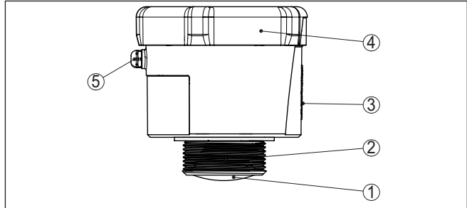
Fig. 1: Composants du capteur VEGAPULS Air 41 - Exemple d'exécution avec filetage G1½
