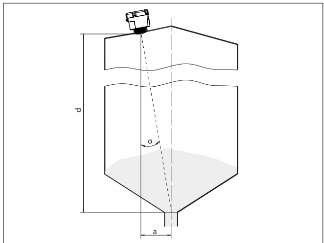
Fig. 12: Proposition pour un montage après orientation VEGAPULS Air 41
