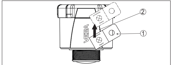
Fig. 14: Activation du capteur par aimant
