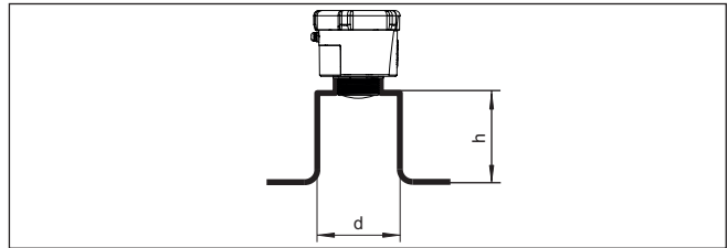
Fig. 9: Montage de la rehausse en cas de dimensions de rehausse différente
