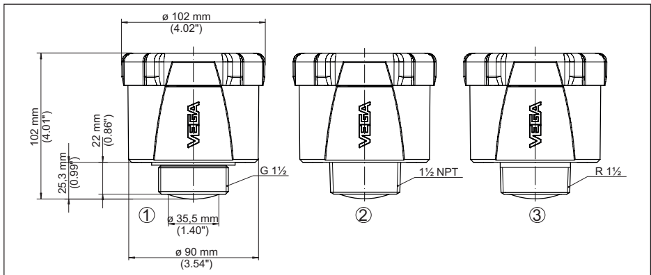
Fig. 29: Encombrement VEGAPULS Air 41
