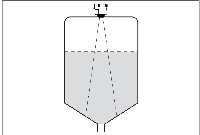
Fig. 6: Montage du capteur radar dans des cuves à fond conique
