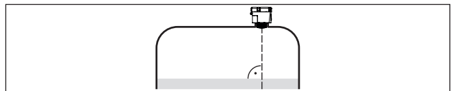
Fig. 10: Orientation du capteur dans les liquides
