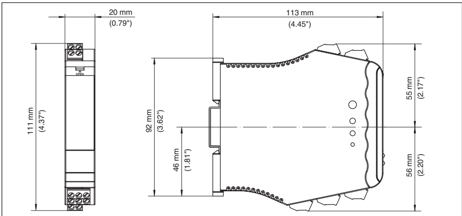
Fig. 2: Medidas VEGATRENN 142
