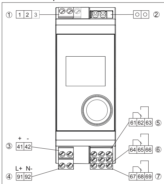
Abb. 3: Anschlussplan VEGAMET 141
