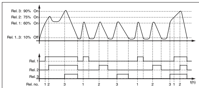
Abb. 15: Beispiel für Pumpensteuerung 4
