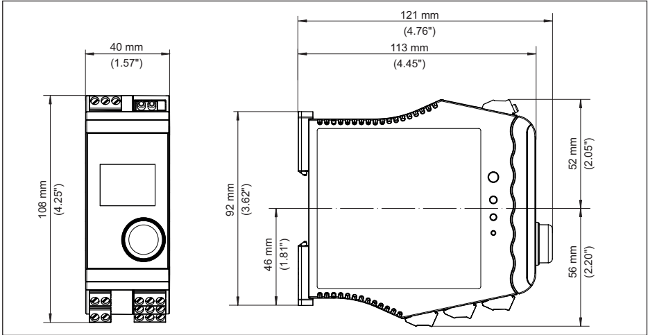
Abb. 19: Maße VEGAMET 141
