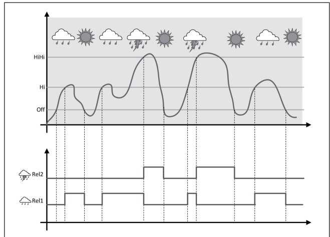
Fig. 14: exemplo de um comando de bombas com a opção "Funcionamento com tempo bom, sem chuva e céu limpo"
