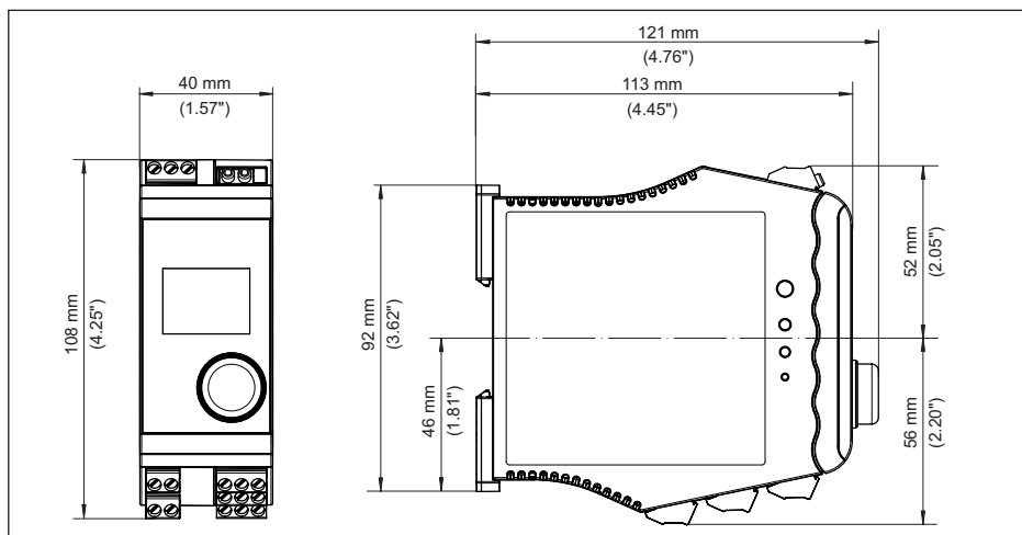
Fig. 19: Dimensões VEGAMET 141
