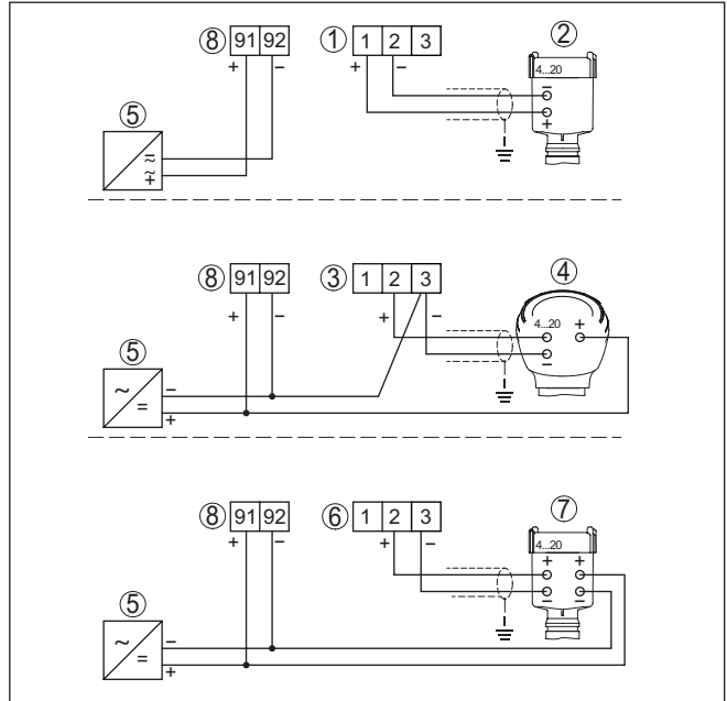
Fig. 4: Conexão sensor de dois/três/quatro condutores (ativo/passivo)
