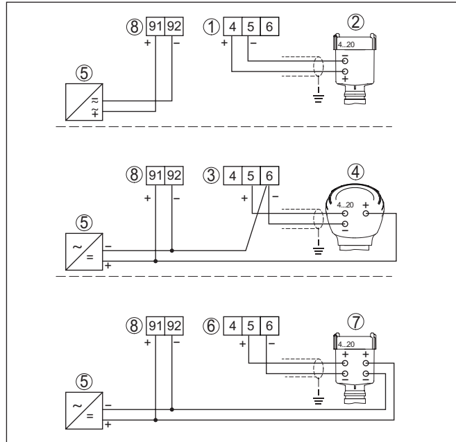
Fig. 5: Conexão sensor de dois/três/quatro condutores (ativo/passivo)
