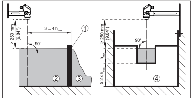
Fig. 19: Medição de débito com vertedouro retangular: h_{máx.} = máx. enchimento da calha retangular
