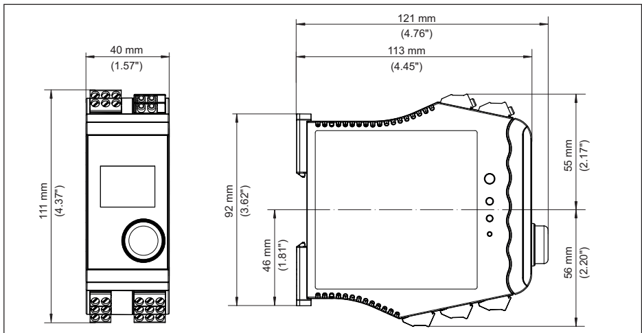
Fig. 21: Dimensões VEGAMET 142
