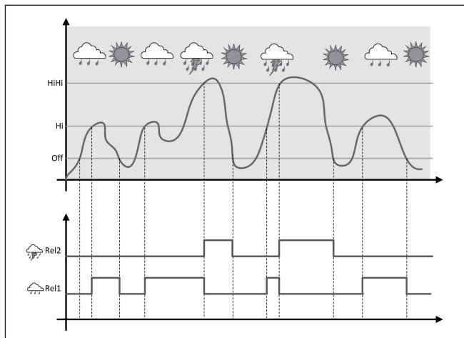
Fig. 15: exemplo de um comando de bombas com a opção "Funcionamento com tempo bom, sem chuva e céu limpo"
