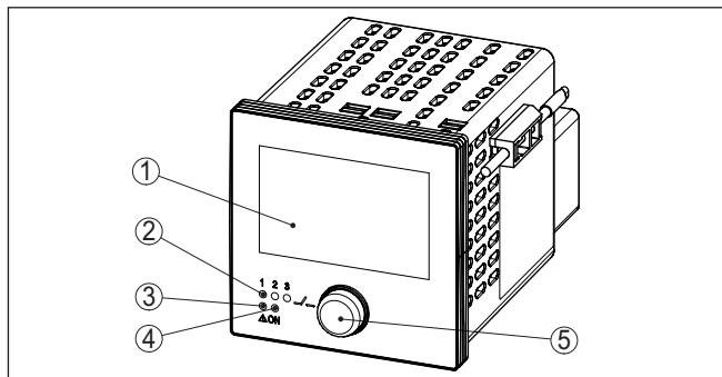
Fig. 7: Aanwijs- en bedieningselementen
