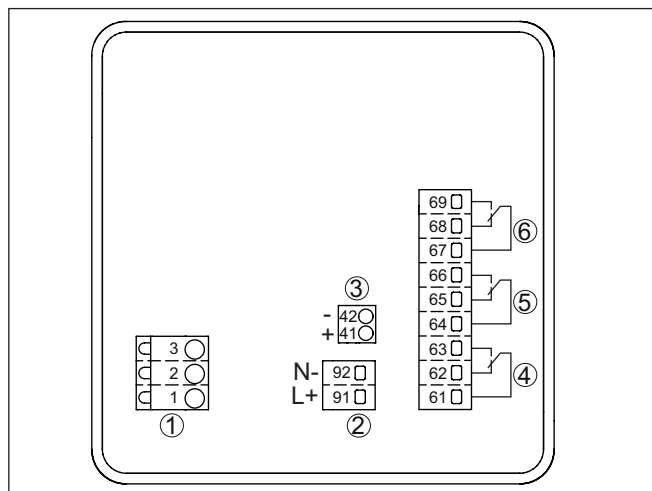
Fig. 4: Aansluitschema VEGAMET 341
