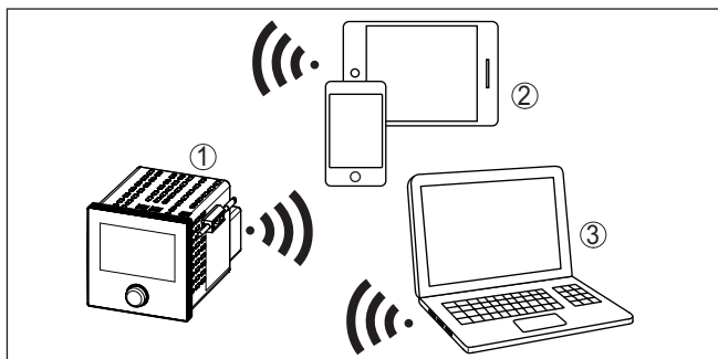
Fig. 2: Draadloze verbinding met standaard bedieningstools met geïntegreerde Bluetooth LE of alternatief Bluetooth-USB-adaptor
