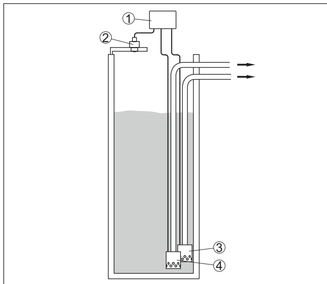
Fig. 13: Voorbeeld pompstation: pompregeling in inlaatschacht
