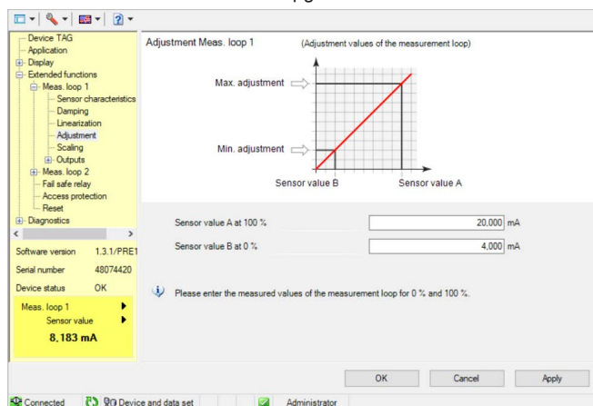
Fig. 11: Voorbeeld van een DTM-aanzicht - Inregeling
