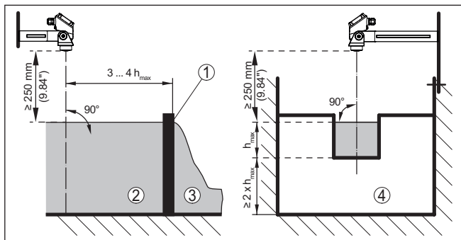
Fig. 19: Flowmeting met rechthoekig overstortschot: h_{\text{max}} = max. vulling van het rechthoekig overstortschot
