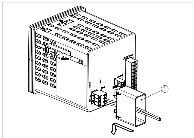
Fig. 6: Plaatsen van de Ex-scheidingskamer
