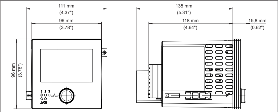
Fig. 21: Afmetingen VEGAMET 341
