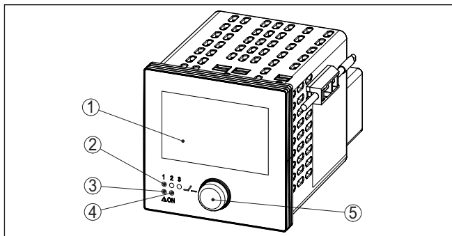
Fig. 8: Aanwijs- en bedieningselementen
