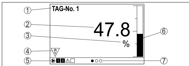
Fig. 9: Voorbeeld meetwaarde-indicatie (meetwaarde met bargraph)
