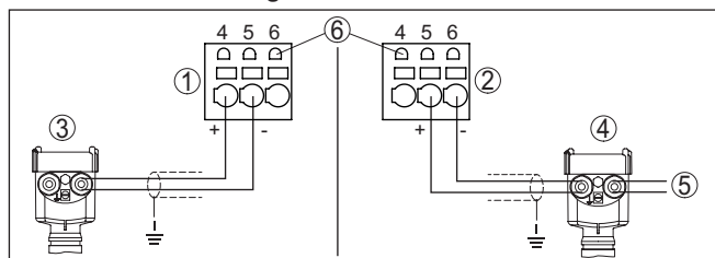
Fig. 6: Aansluiting ingang 2 voor tweedraads-/vierdraadssensor (actief/passief)
