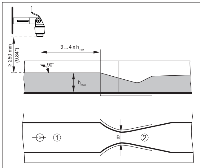
Fig. 22: Flowmeting met Khafagi-venturigoot: h_{max} = max. peil in de goot; B = maximale insnoering van de goot
