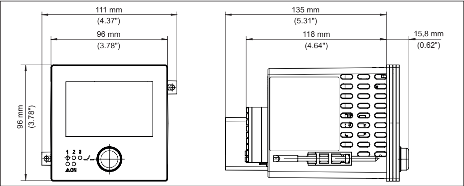
Fig. 23: Afmetingen VEGAMET 342
