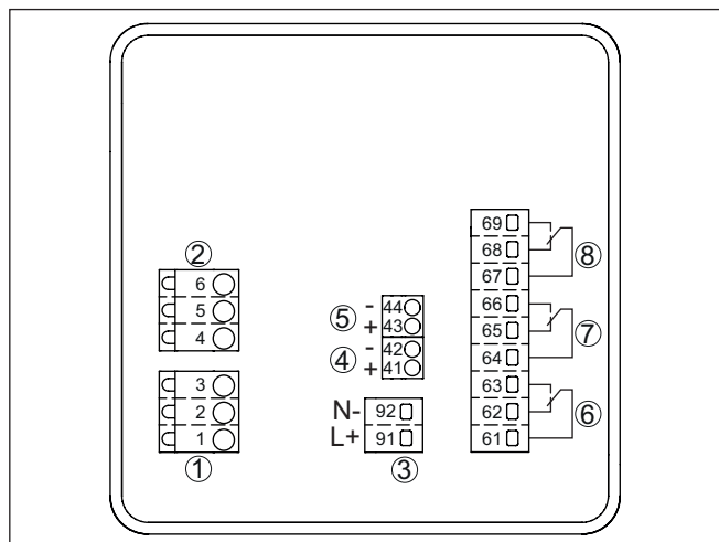
Fig. 4: Aansluitschema VEGAMET 342
