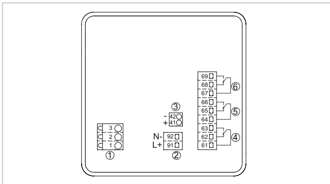
Schema di collegamento VEGAMET 341
